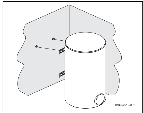
Fig. 8 Instalación vertical (montaje en pared)
