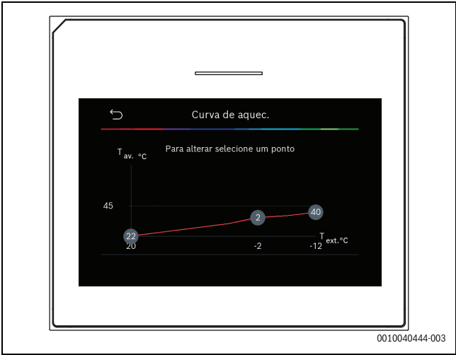
Fig. 1 Ecrã inicial para ajustar a curva de aquecimento para o tipo de regulação da temperatura exterior com ponto de funcionamento (e ponto de conforto)
