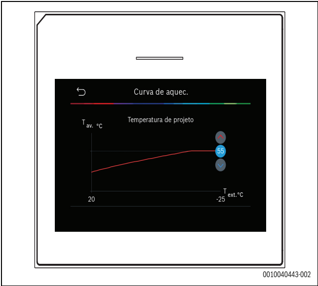
Fig. 2 Ajuste o ponto final (apenas se o tipo de controlo estiver definido para temperatura exterior com ponto de funcionamento)
