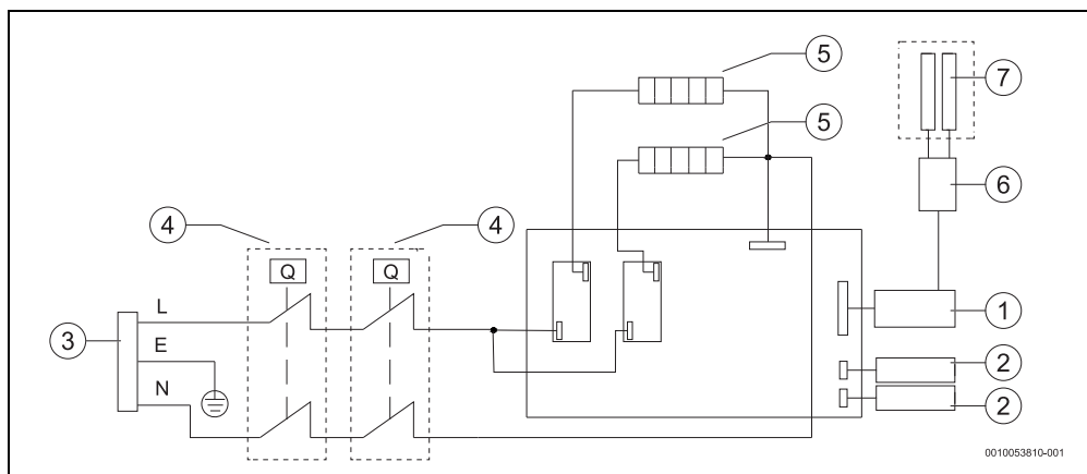
Bild 17 Anschlusschema
