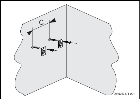
Bild 10 Montageplatten
