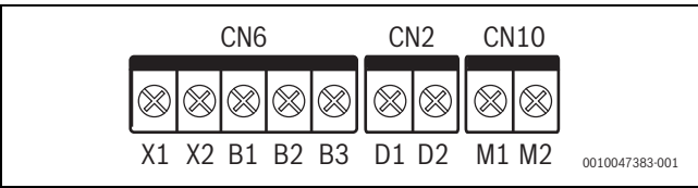
Fig. 24 Terminal de comunicare
