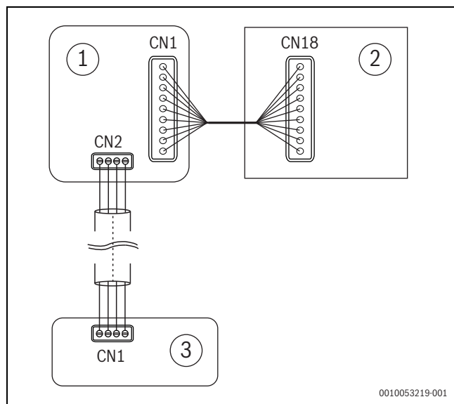
Sl.32 Senzor curenja jedan/dva
