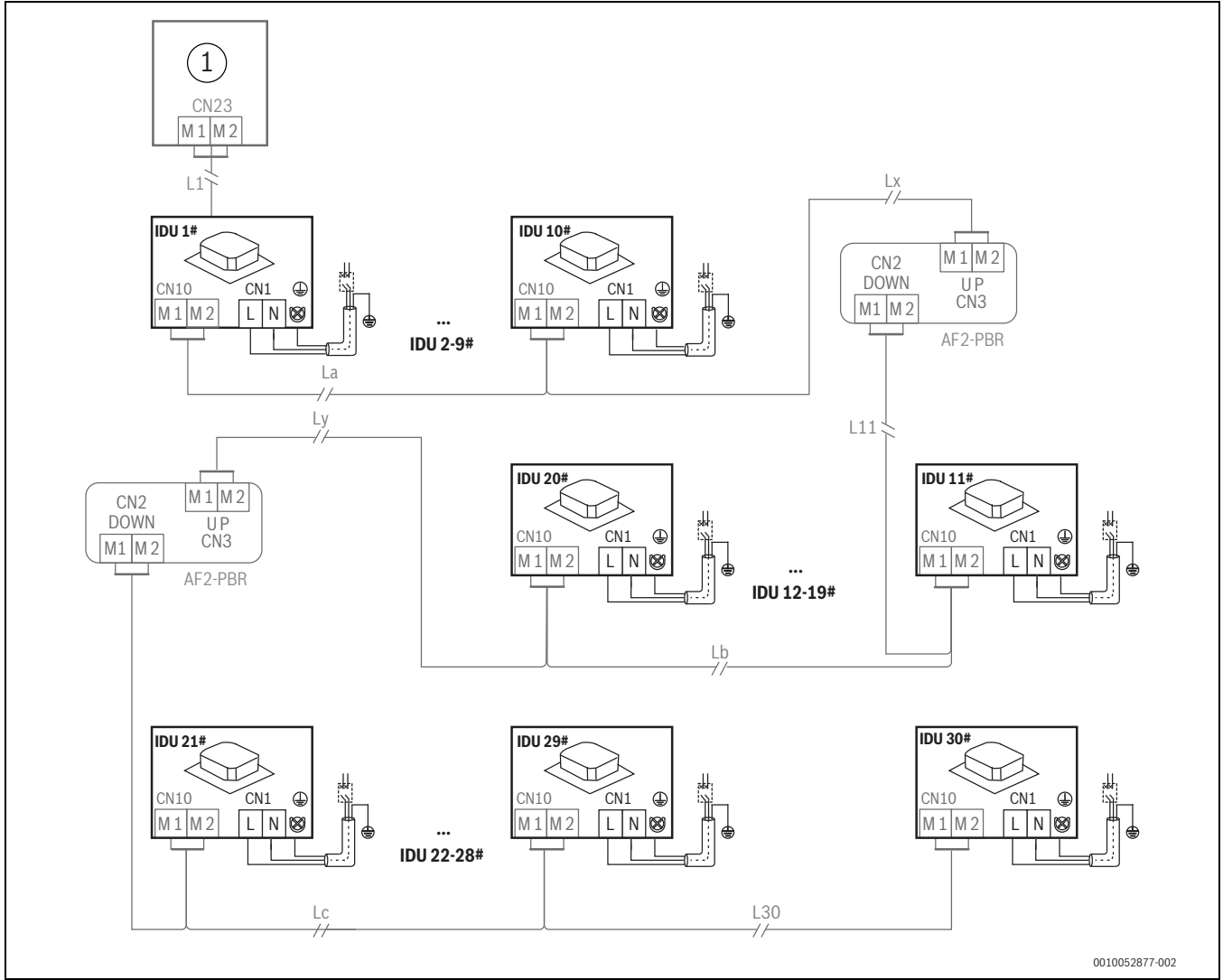
Res. 25 İç ve dış üniteler iletişim kablosu (M1/M2), bağımsız güç kaynağı ile
