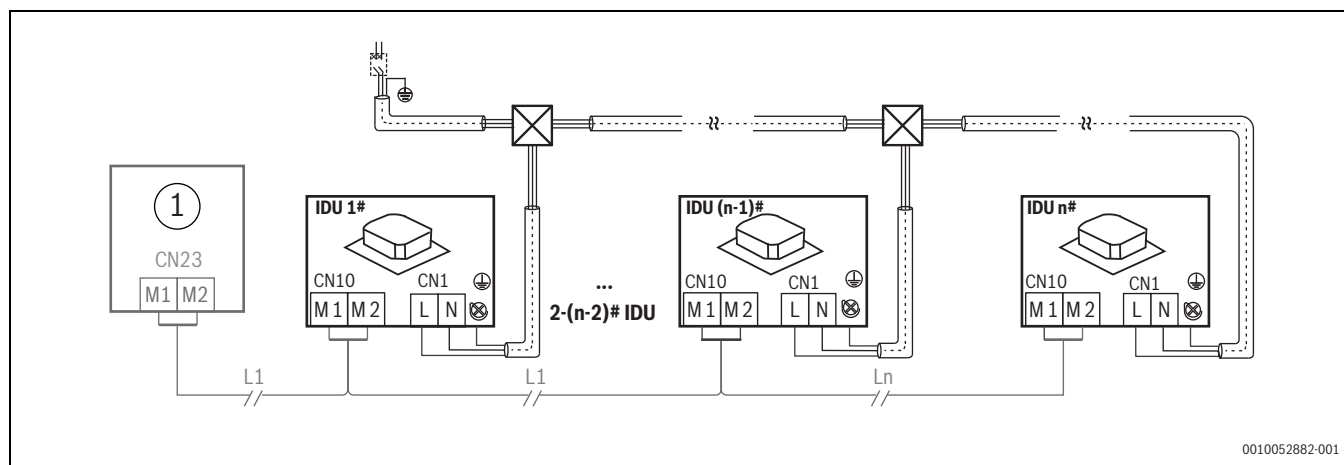
Sl.26 Komunikacijsko ožičenje unutarnjih i vanjskih jedinica (M1/M2) s ujednačenim napajanjem
