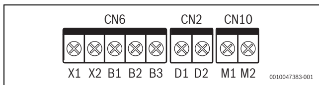
SI.24 Komunikacijska priključna stezaljka
