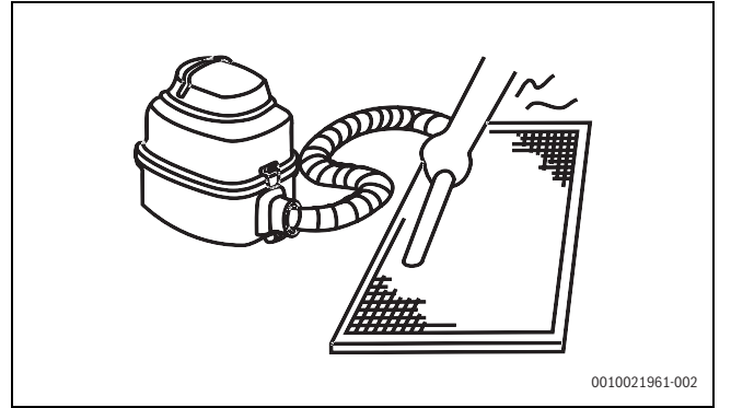
Res. 39 Hava giriş ağzının elektrikli süpürgeyle temizlenmesi
