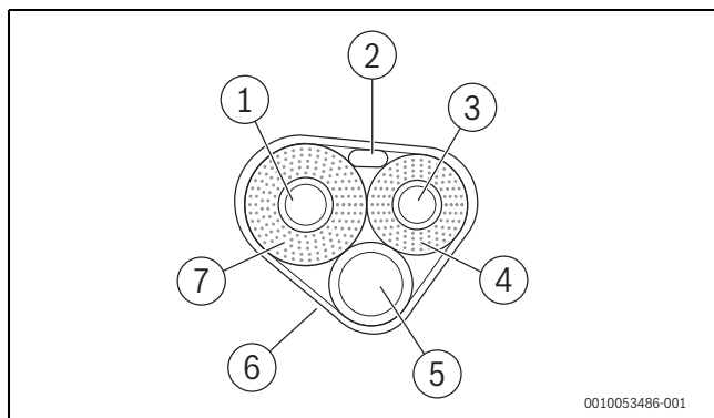
Fig. 16 Isolamento do tubo
