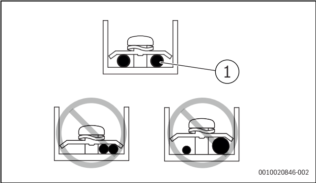
Fig. 21 Ligações do cabo de alimentação, corretas e incorretas
