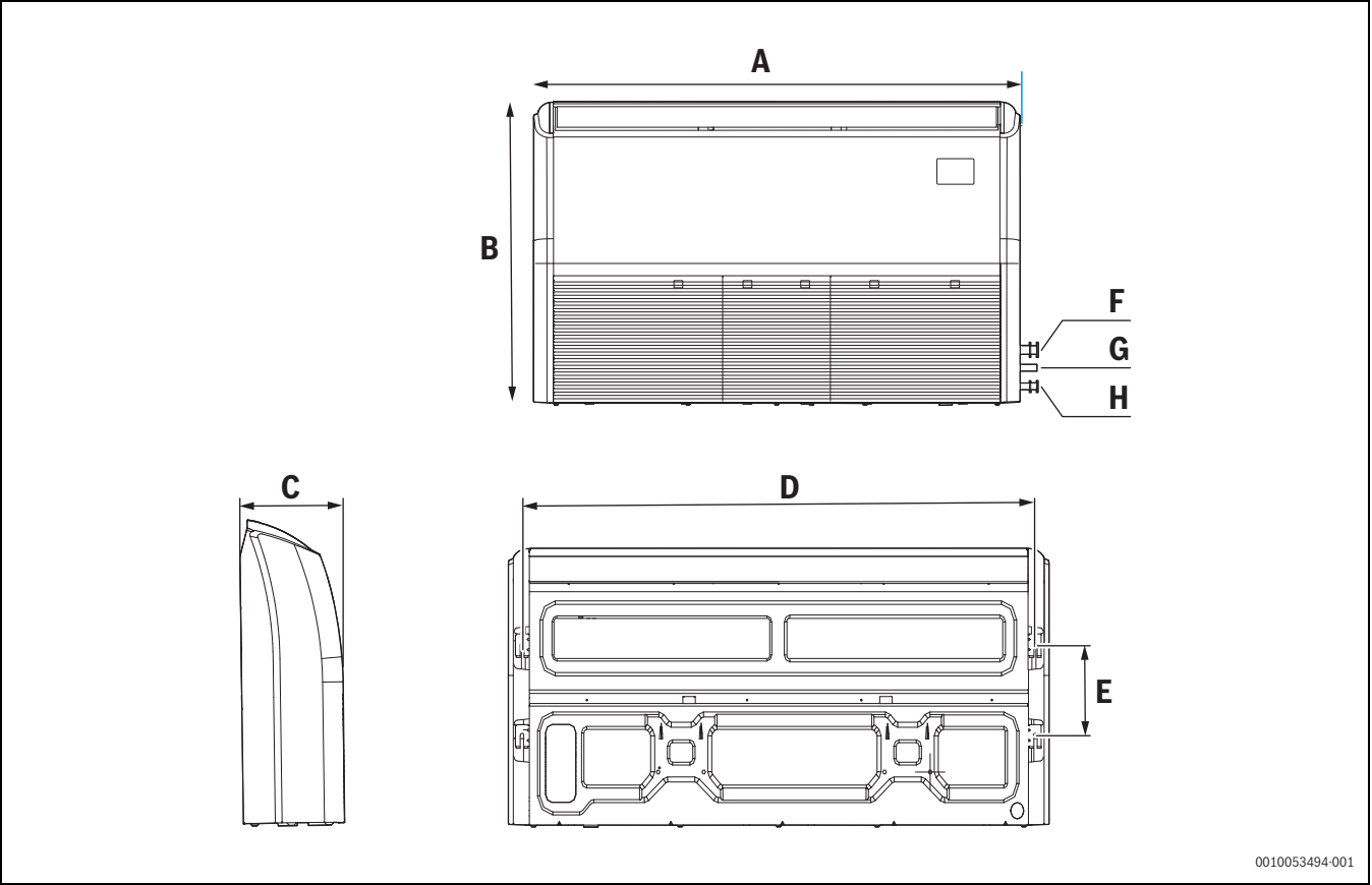
Fig. 5 Dimensiuni externe și mărimea orificiului pentru evacuarea aerului (unitate: mm)
