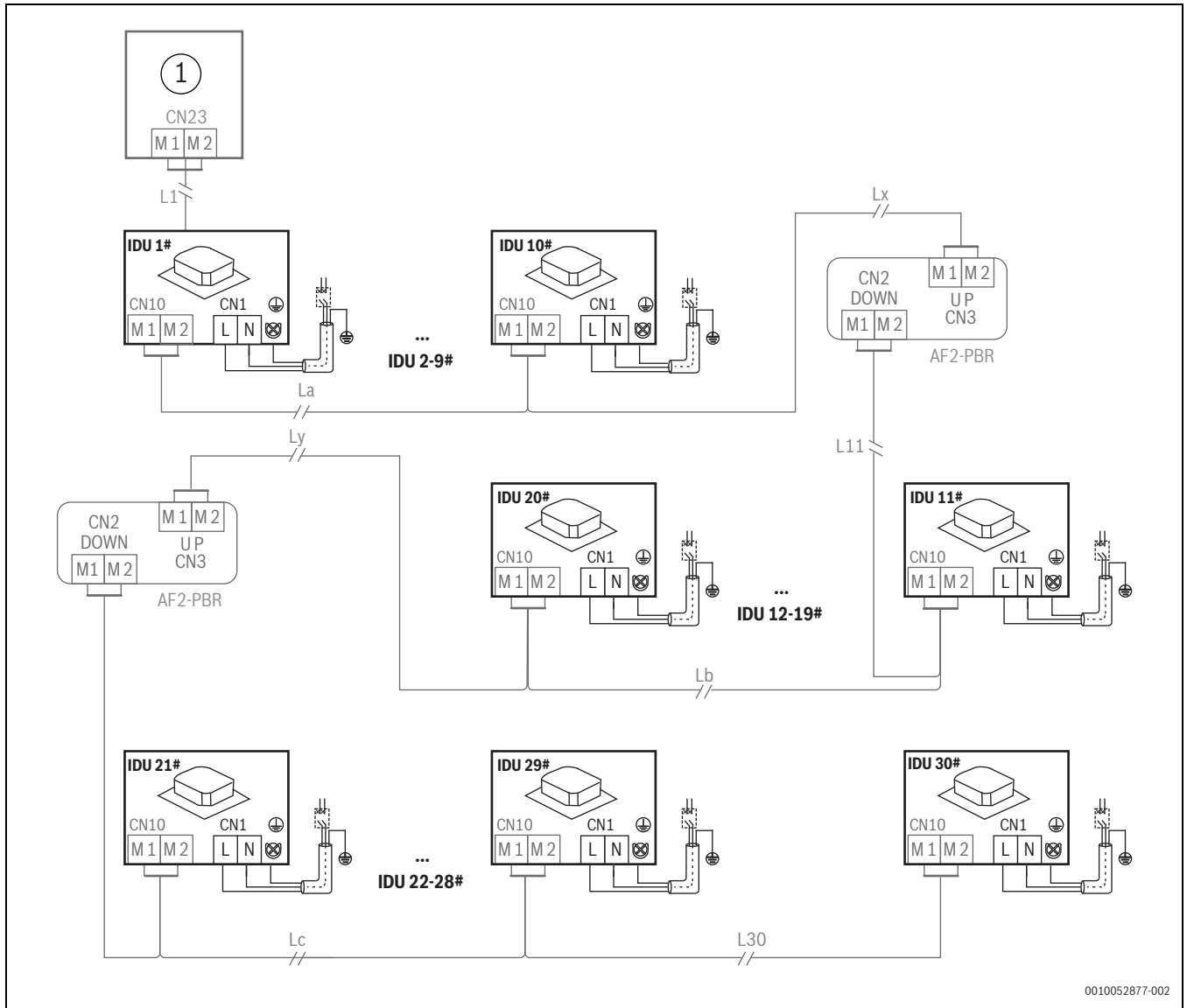
Fig. 25 Cabo de comunicação das unidades interior e exterior (M1/M2) com alimentação elétrica independente
