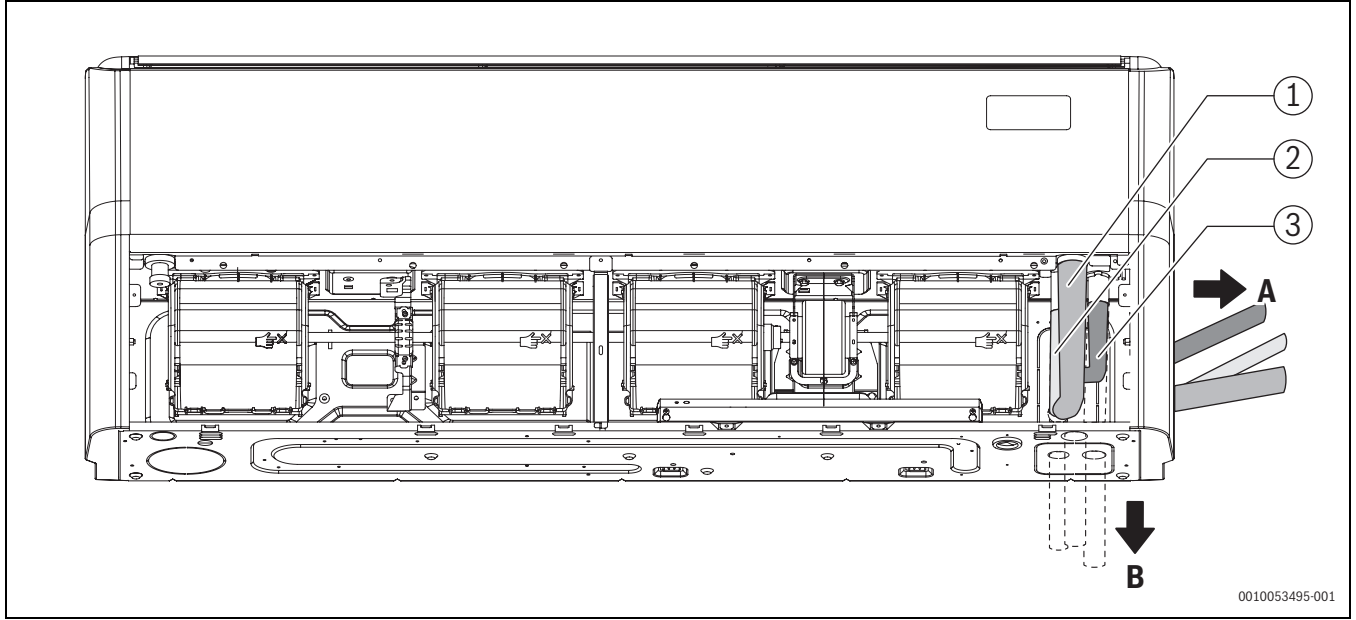
Res. 6 Soğutucu akışkan ve tahliye borularını döşeme yönü.
