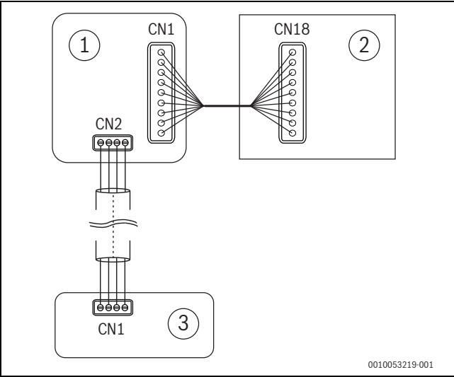
Fig. 32 Senzor de scurgeri unu/doi
