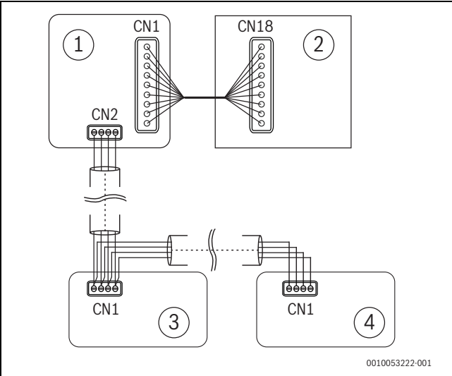
Fig. 33 Senzor de scurgeri unu și doi
