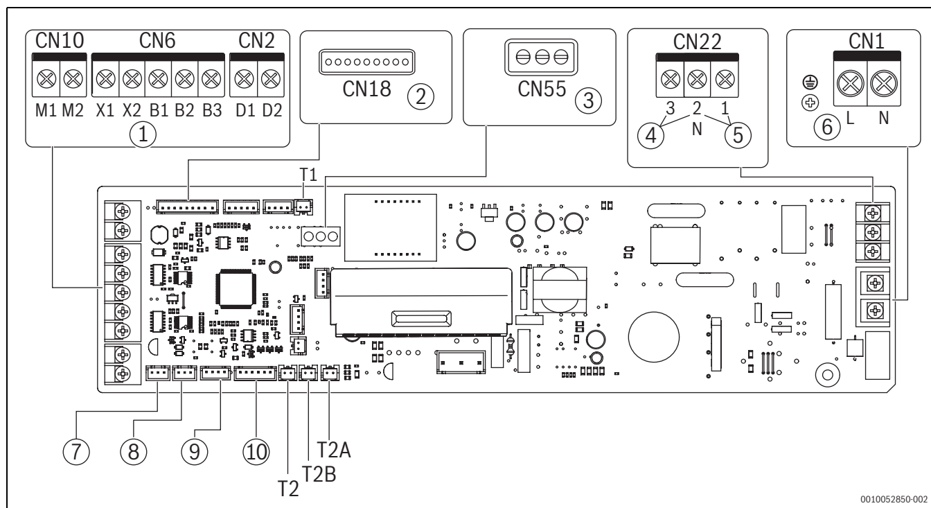
Fig. 50 Schemă electrică utilizator
