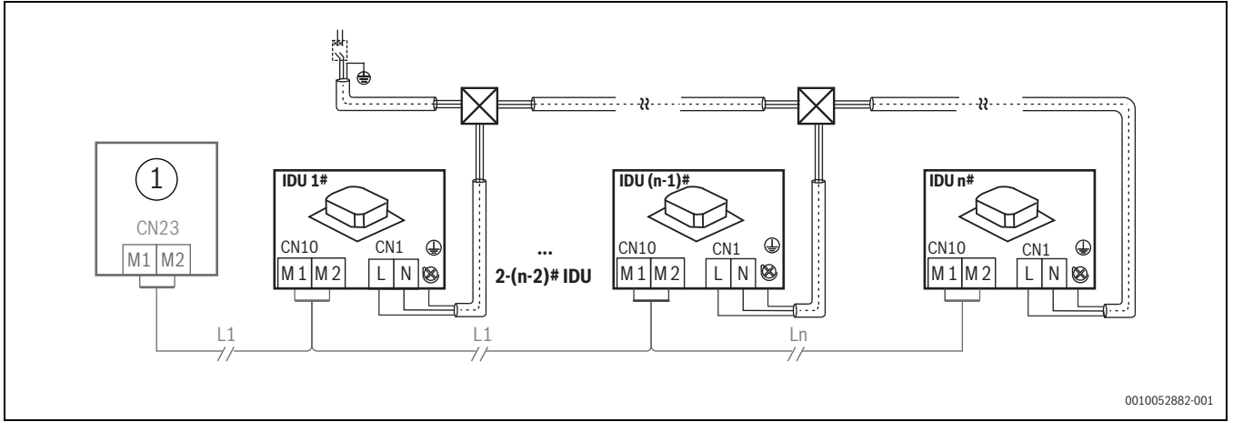
Res. 26 İç ve dış üniteler iletişim kablosu (M1/M2), düzenli güç kaynağı ile
