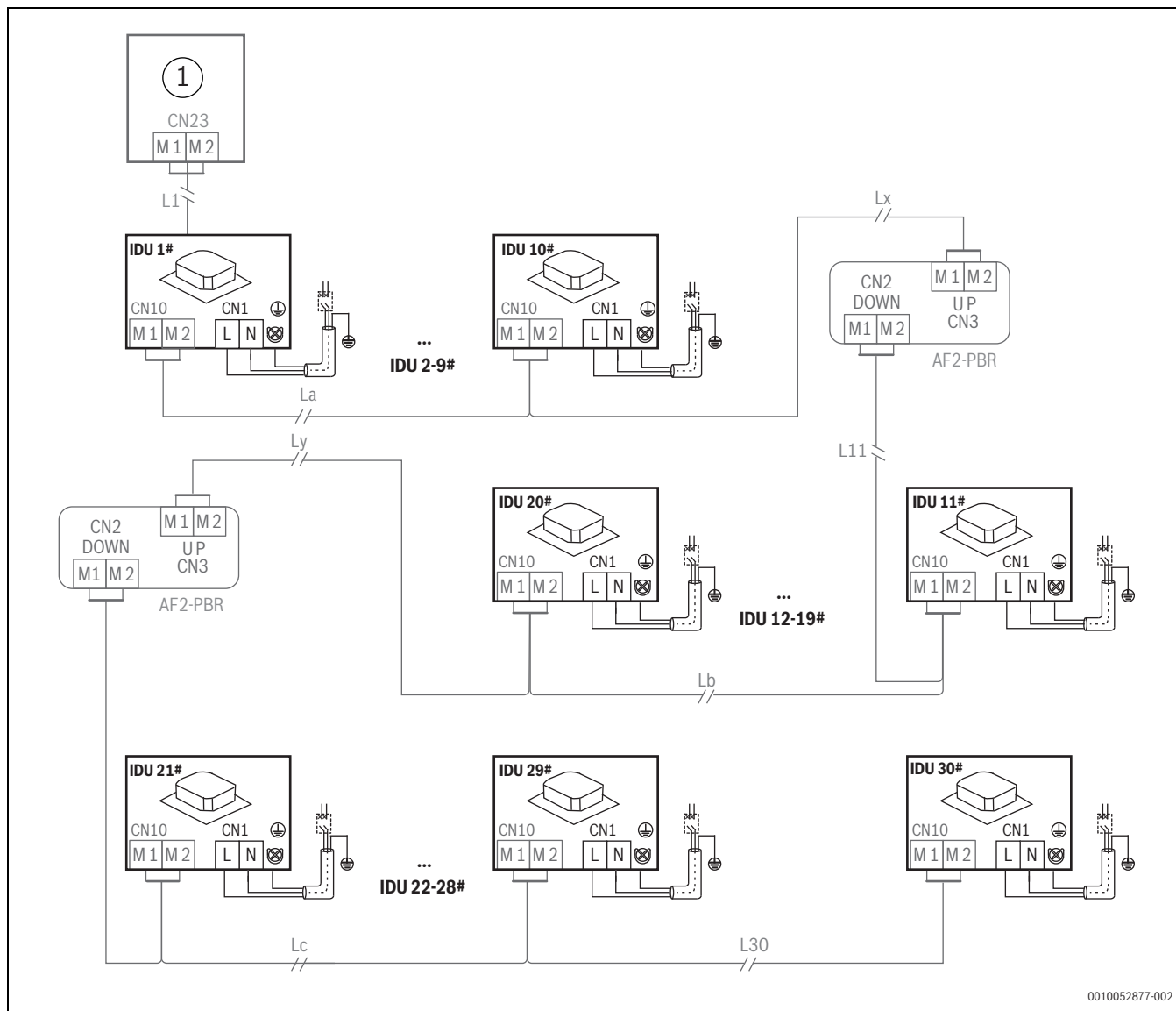
Sl.25 Komunikacijsko ožičenje unutarnjih i vanjskih jedinica (M1/M2) s nezavisnim napajanjem
