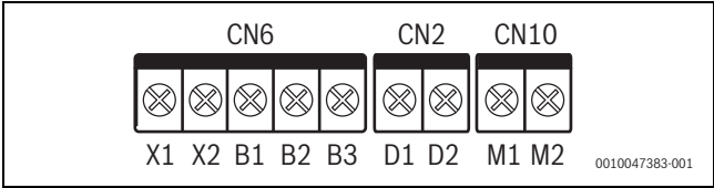
Fig. 24 Terminal de comunicação
