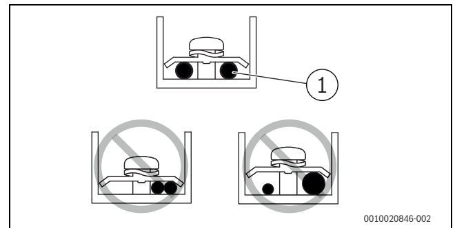
Res. 21 Doğru ve yanlış güç kablosu bağlantıları
