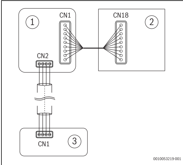
Res. 32 Kaçak sensörü bir/iki
