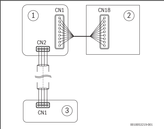
Fig. 32 Sensor de fuga um/duos
