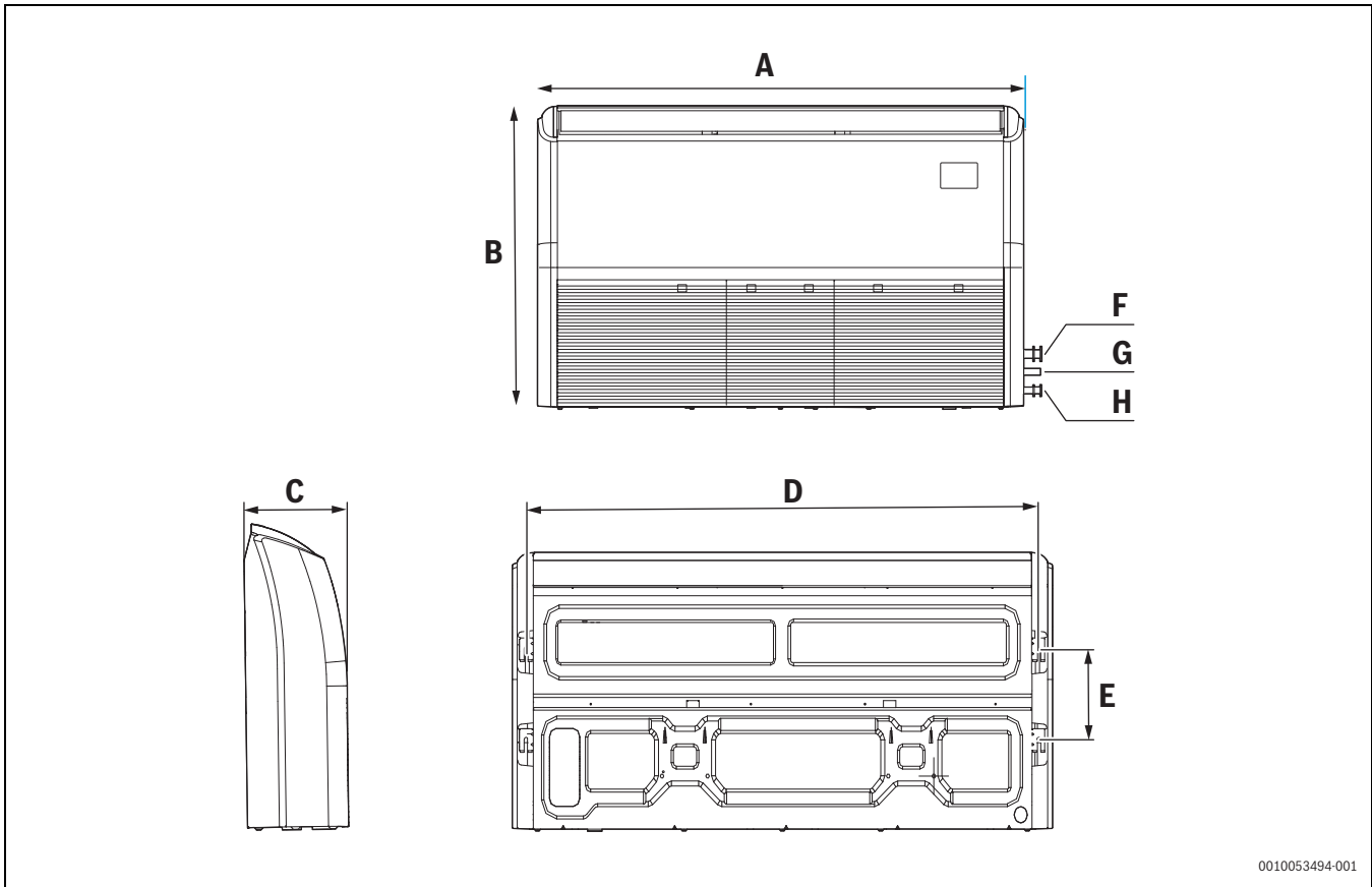
Sl.5 Vanjske dimenzije i veličina otvora izlaza zraka (jedinica: mm)
