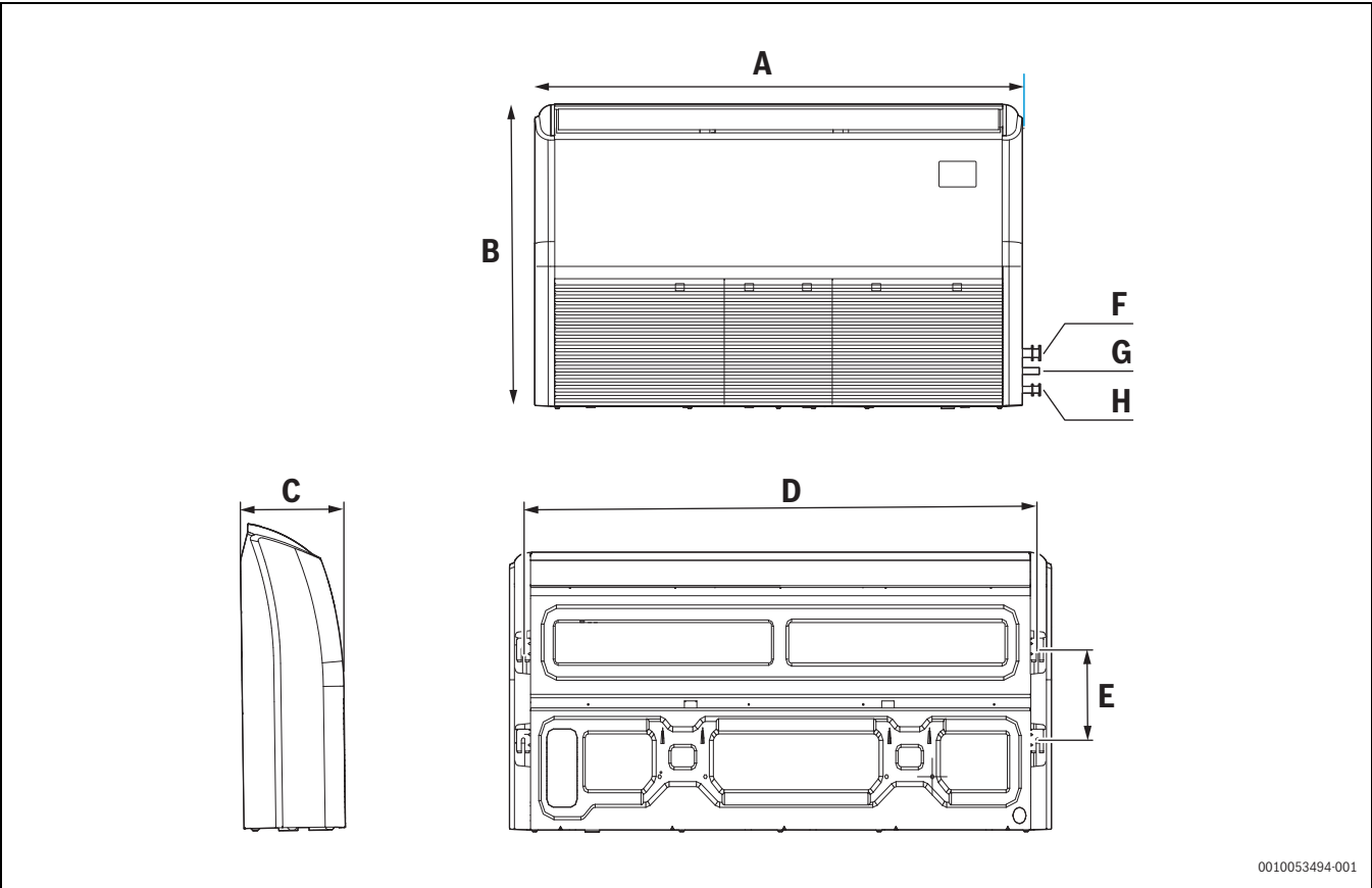
Fig. 5 Dimensões do corpo e da abertura de saída de ar (unidade:mm)
