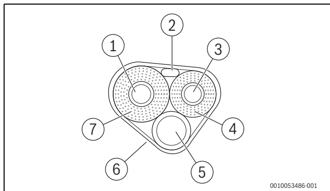
Fig. 16 Izolarea țevilor
