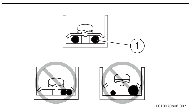
Sl.21 Pravilni i nepravilni priključci ožičenja napajanja
