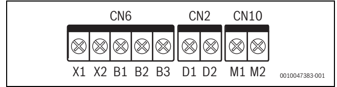
Res. 24 İletişim terminali
