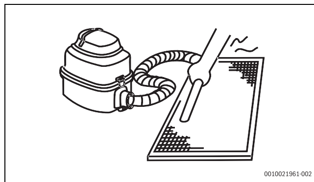
SI.39 Čišćenje ulaza zraka usisivačem
