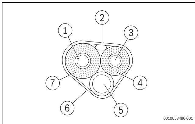
Sl. 16 Izolacija cjevovoda
