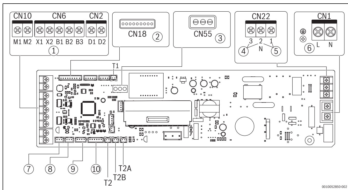
Sl.50 Korisnikova shema spajanja
