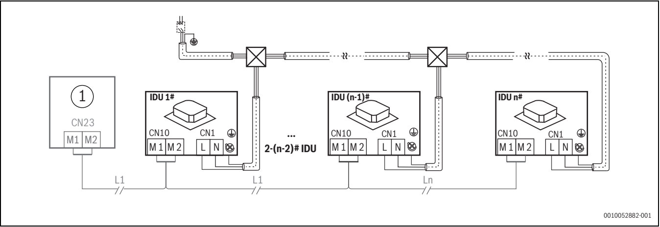
Fig. 26 Cabo de comunicação das unidades interior e exterior (M1/M2) com alimentação elétrica uniforme
