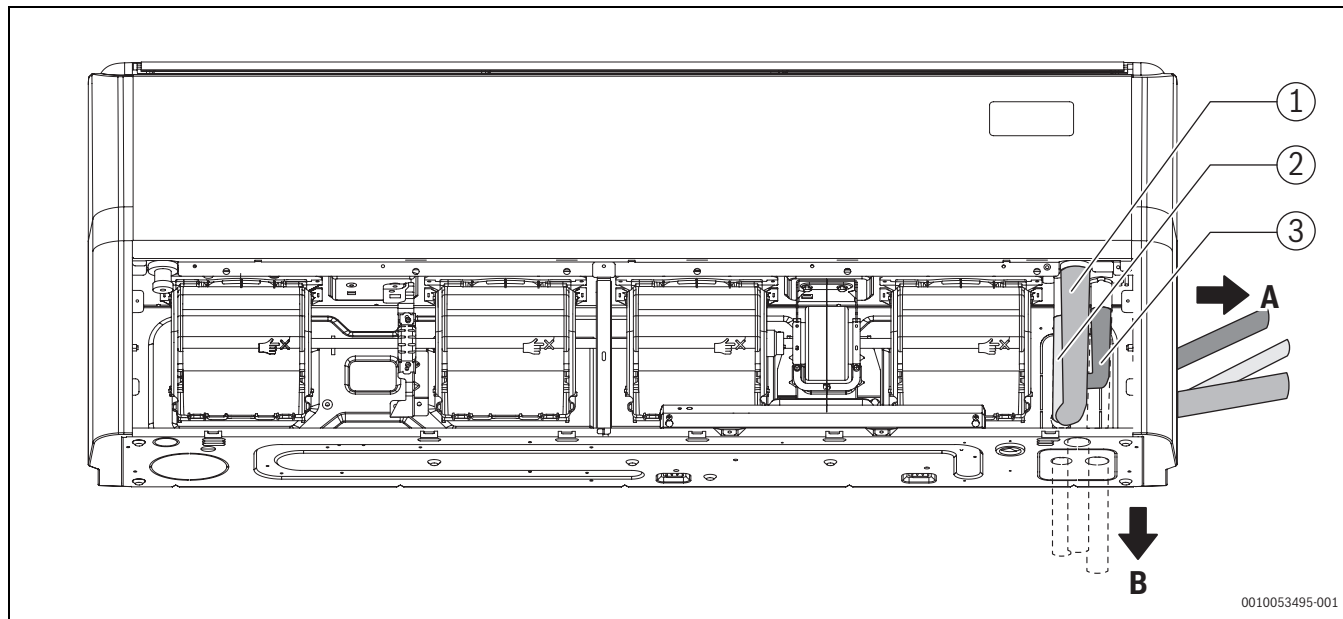
Sl.6 Smjer polaganja cijevi rashladnog sredstva i odvodnih cijevi.
