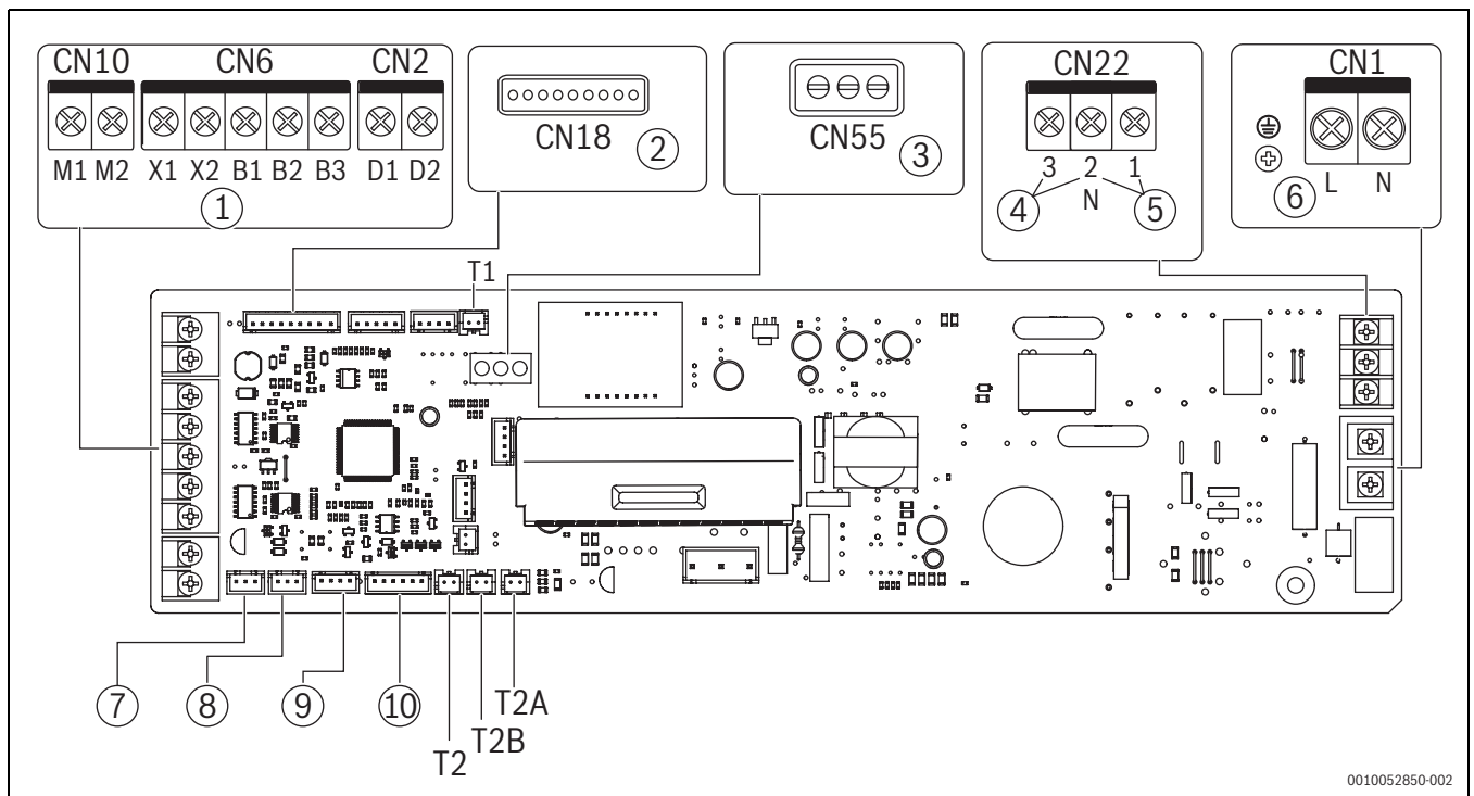
Fig. 50 Esquema elétrico do utilizador
