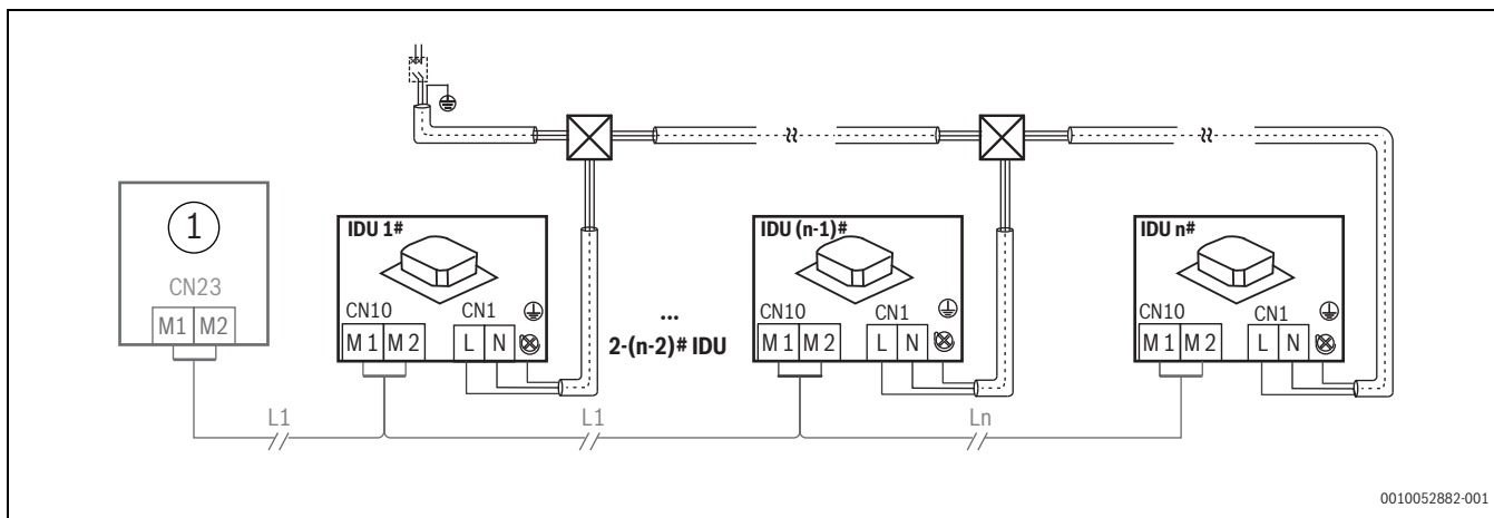
Fig. 26 Cablu de comunicare între unitățile interioare și externe (M1/M2) cu alimentare cu energie electrică uniformă
