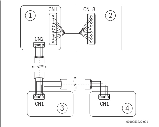
Fig. 33 Sensor de fuga um e dois
