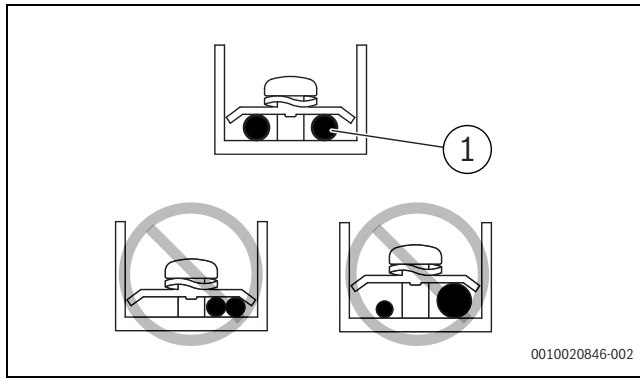
Fig. 21 Conexiuni de cablare corespunzătoare și necorespunzătoare
