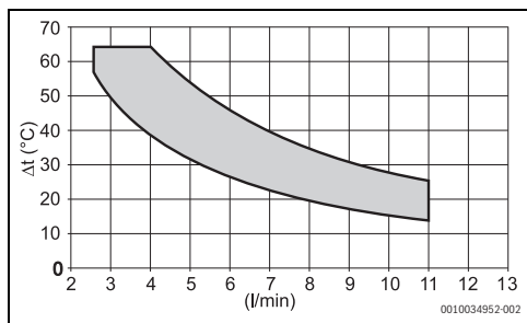
Fig. 31 Modelo 11 litros
