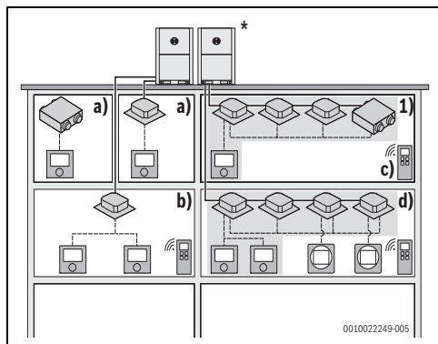
Fig. 1 Casos de aplicação de ARC C-2/ARC H-2 (visão esquemática; a figura não mostra a cablagem/sistema de tubagens real)
