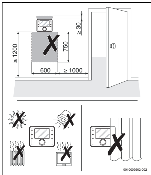
Fig. 4 Local de instalação na zona de referência
