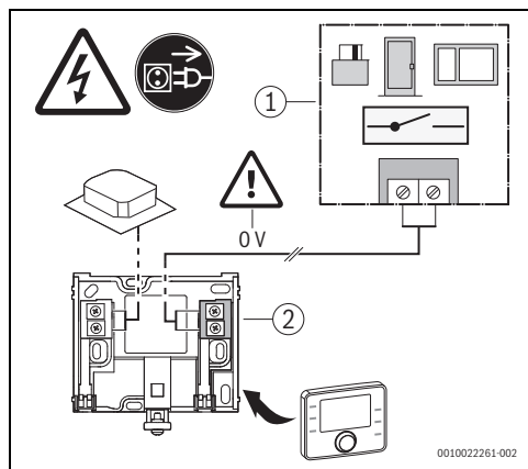
Fig. 7 Ligação do interruptor de contacto à unidade de comando ARC H-2
