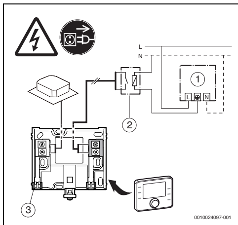
Fig. 8 Ligação de um interrupor com tensão (exemplo)
