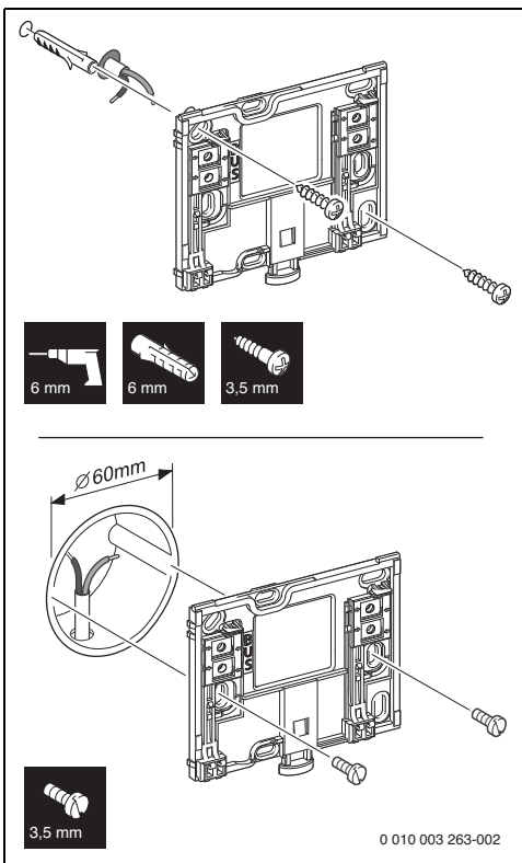
Fig. 5 Montagem da base de parede
