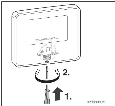
Fig. 10 Aparafusar/Desaparafusar o parafuso de fixação
