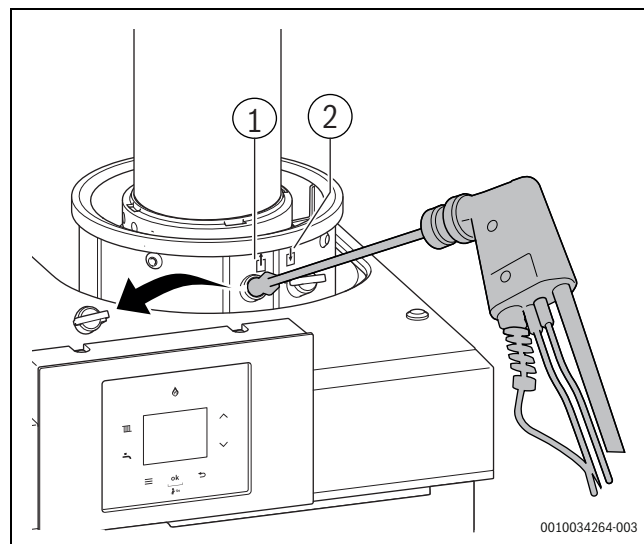
Fig. 34 Remova o tampão na saída de gases queimados
