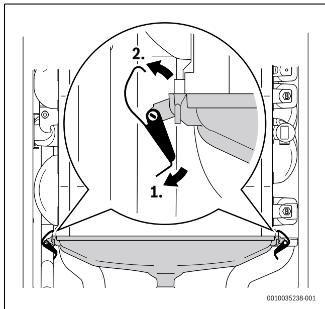
Fig. 45 Abra o fecho com mosquetão da cuba de condensados
