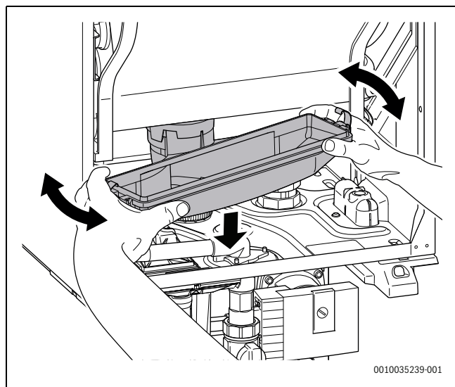
Fig. 46 Remova a cuba de condensados.
