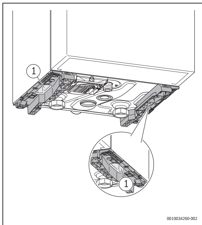
Fig. 7 Posição das depressões da pega
