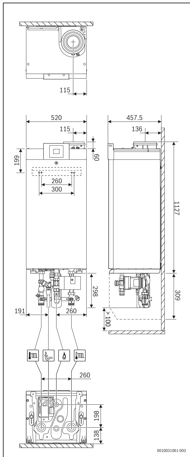
Fig. 3 Dimensões na parede [mm]
