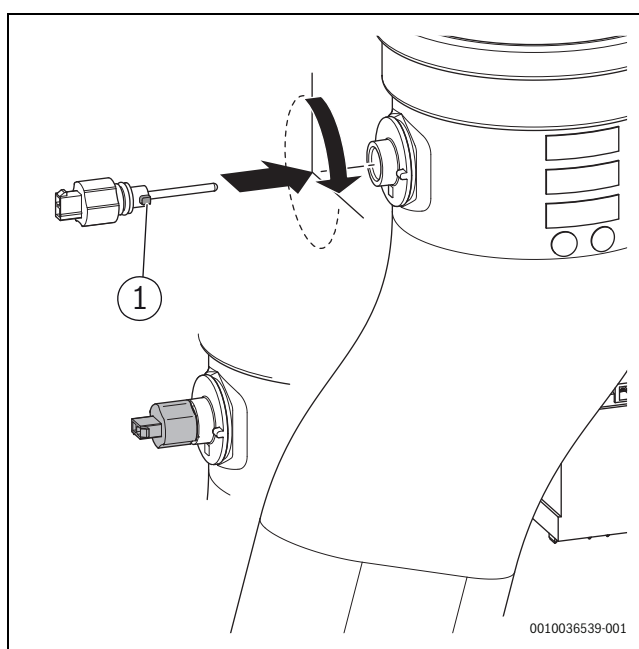
Fig. 48 Substituição do sensor de temperatura dos gases queimados
