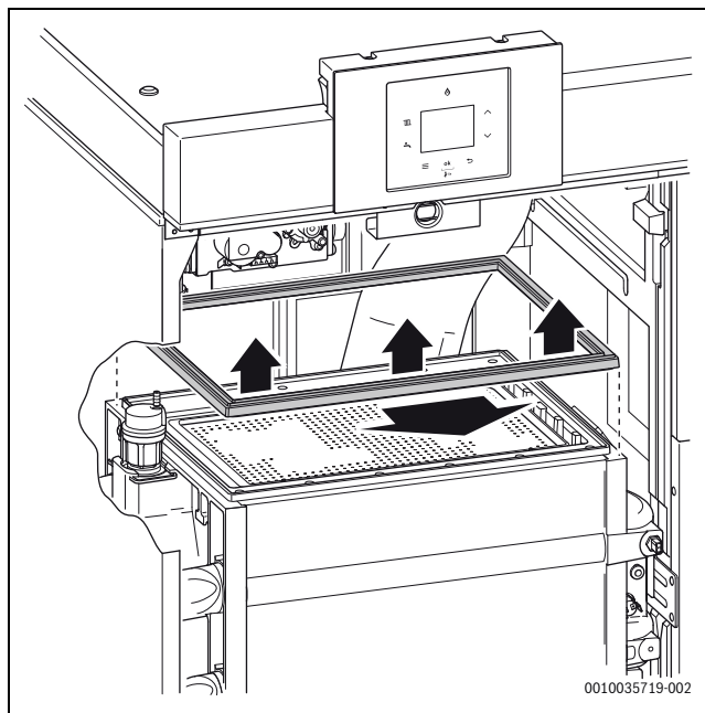
Fig. 41 Remover a vedação do queimador
