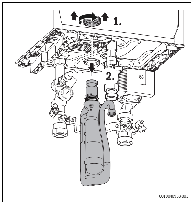
Fig. 44 Remova o sifão da caldeira
