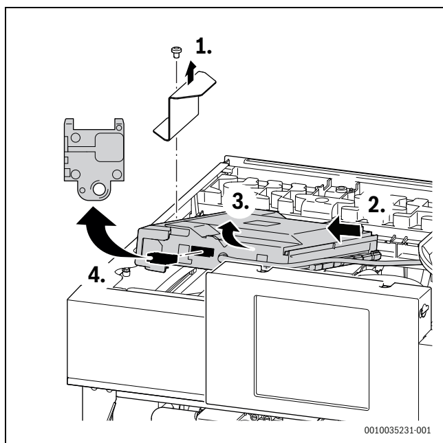
Fig. 49 Substituir a ficha de codificação
