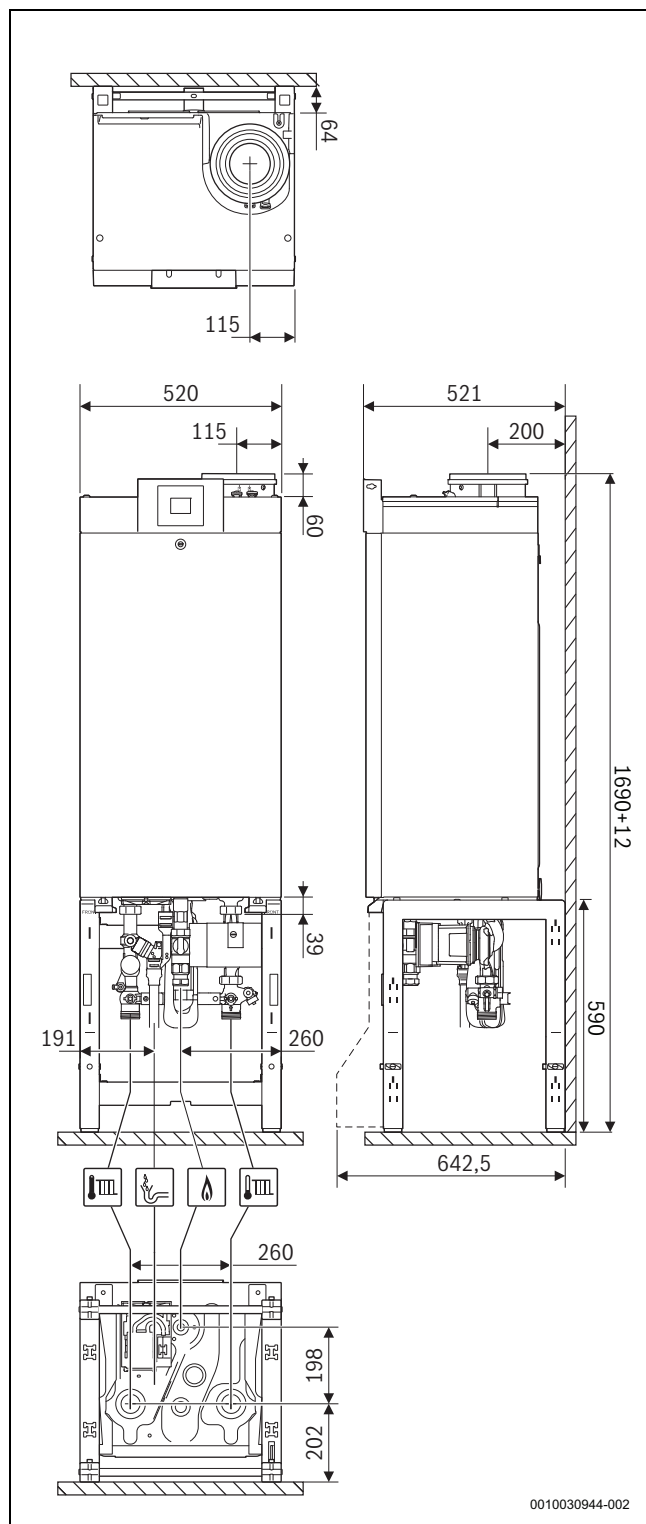
Fig. 2 Dimensões na estrutura de base [mm]
