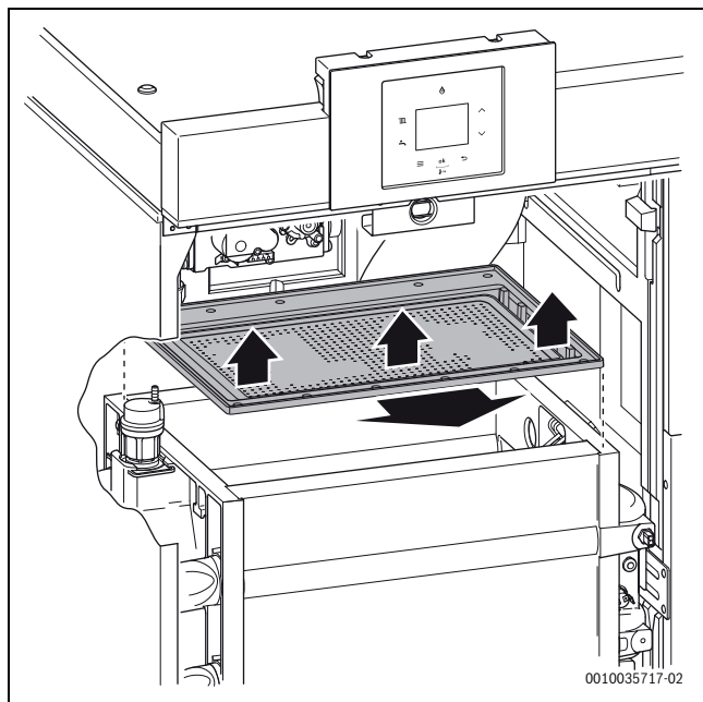
Fig. 42 Desmontar o queimador
