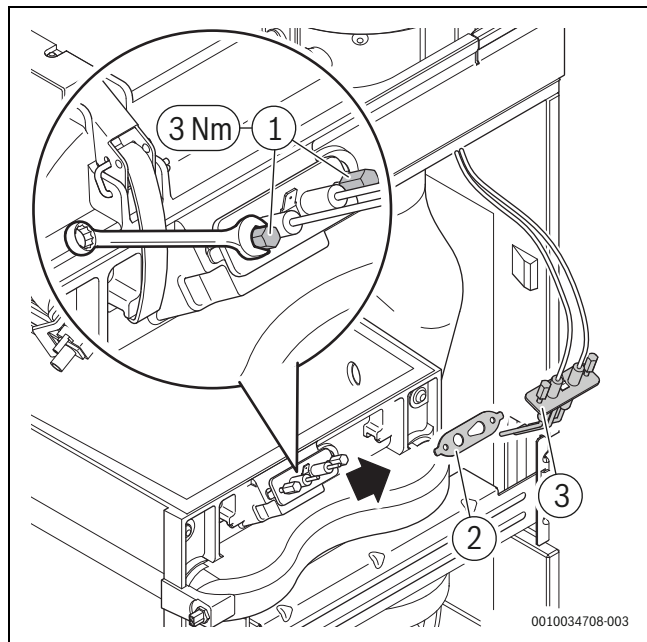
Fig. 47 Inserir o acendedor
