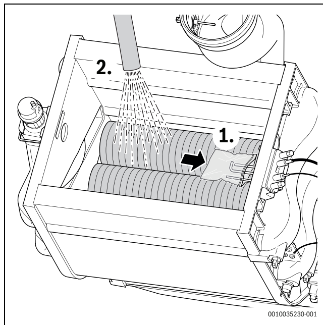
Fig. 43 Limpar o permutador de calor
