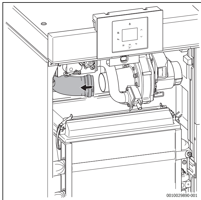
Fig. 38 Remover a conduta de admissão de ar
