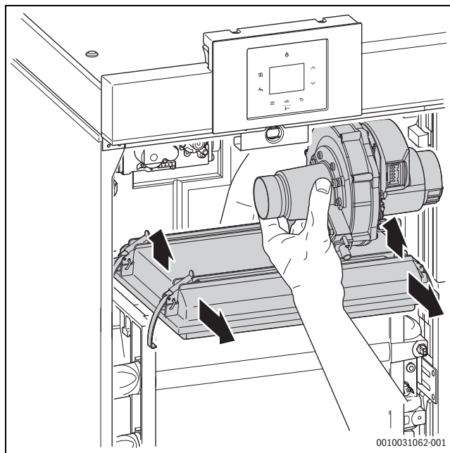
Fig. 40 Remova a unidade de gás/ar juntamente com a cobertura do queimador.
