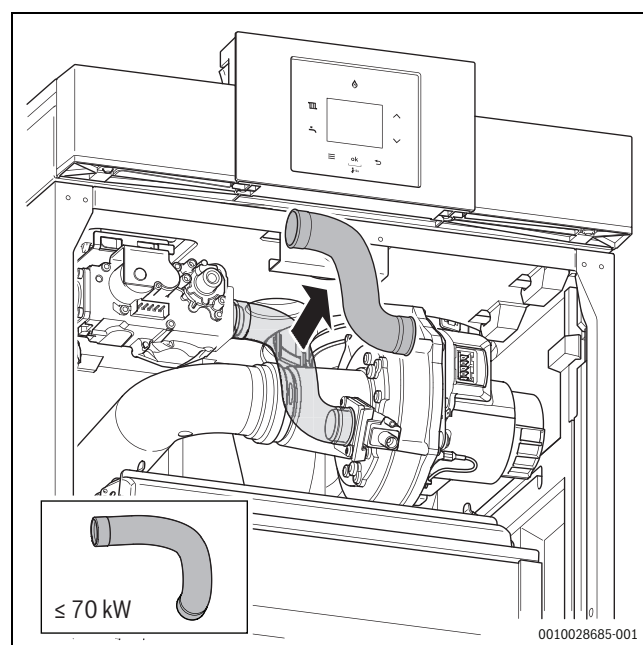
Fig. 37 Remova a mangueira de gás ≥ 85 kW
