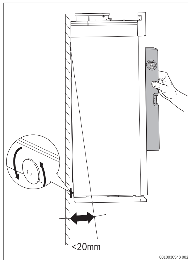
Fig. 12 Alinhar a caldeira na parede
