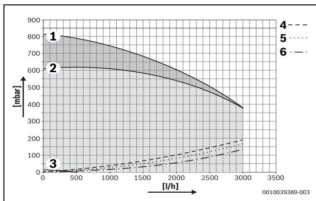
Fig. 51 Altura manométrica residual da bomba GC7000WP 50
