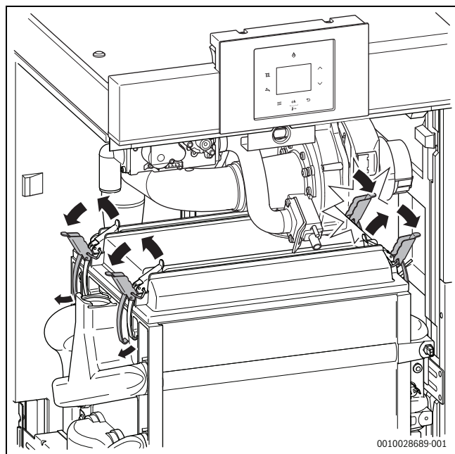
Fig. 39 Abra os fechos com mosquetão
