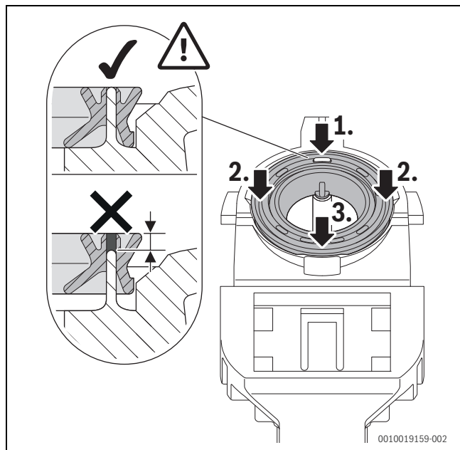
Fig. 59 Pressionar a vedação
