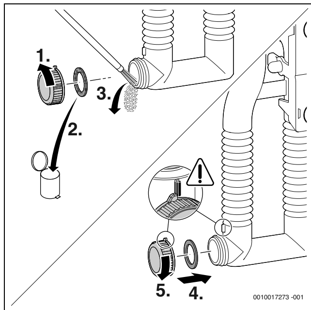
Fig. 56 Limpar a recolha de condensados
