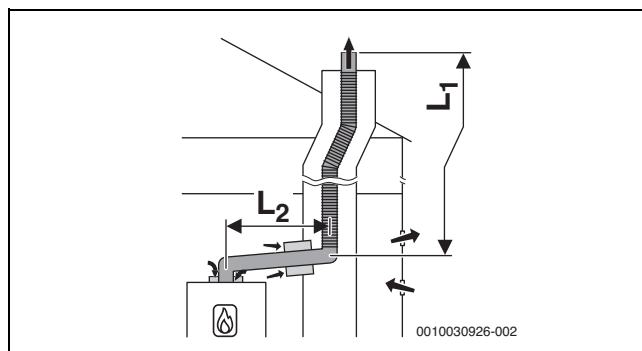
Fig. 13 Tubagem flexível de gases queimados na conduta de acordo com B 23p /B 53p com ar de admissão dependente do ar ambiente no aparelho e peça de ligação concêntrica entre o local de instalação e a conduta
