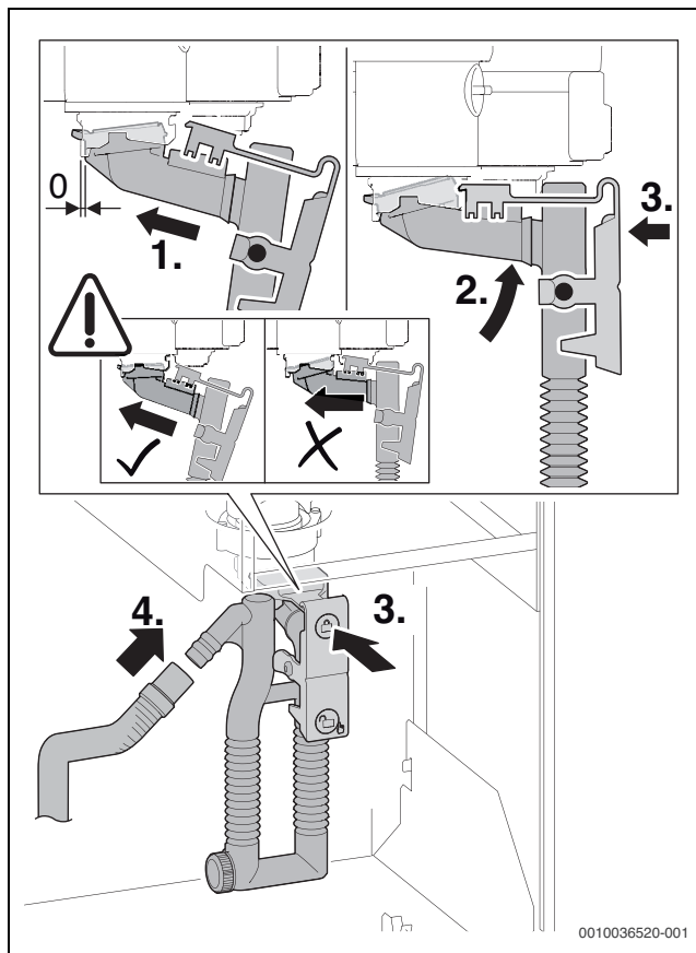
Fig. 60 Instalar a recolha de condensados
