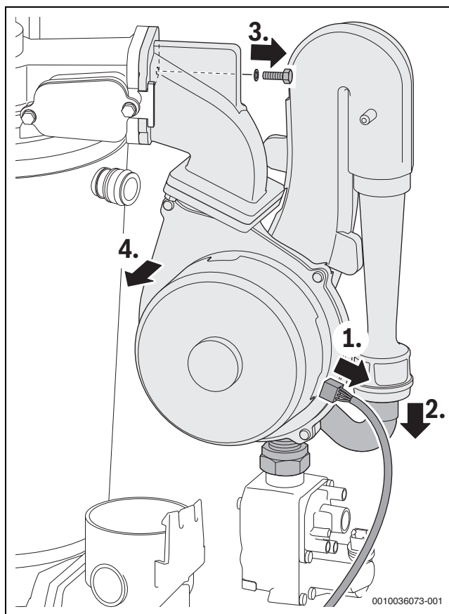
Fig. 44 Desmontar o ventilador com dispositivo de mistura
