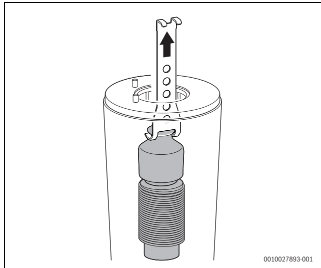
Fig. 48 Retirar o corpo de deslocamento superior
