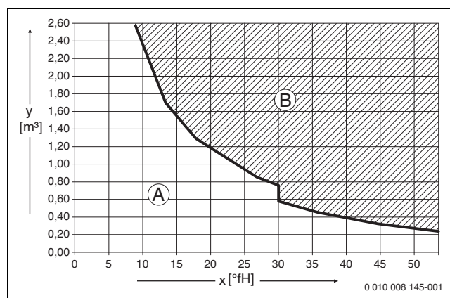
Fig. 15 Requisitos relativos à água de enchimento e à água adicional em °fH para instalações < 50 kW
