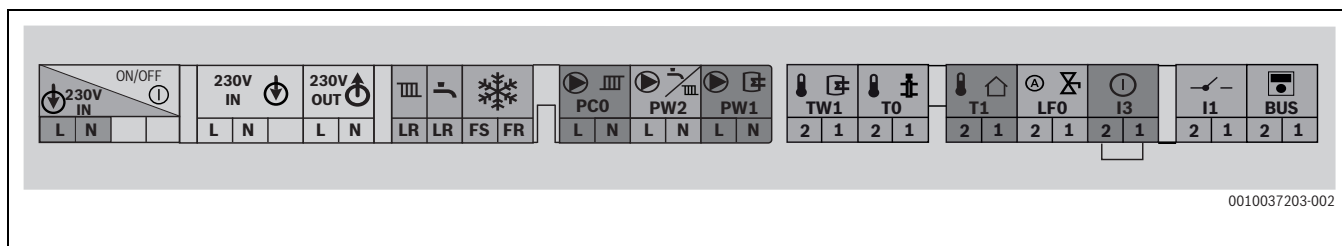
Fig. 31 Régua de bornes para os acessórios externos
