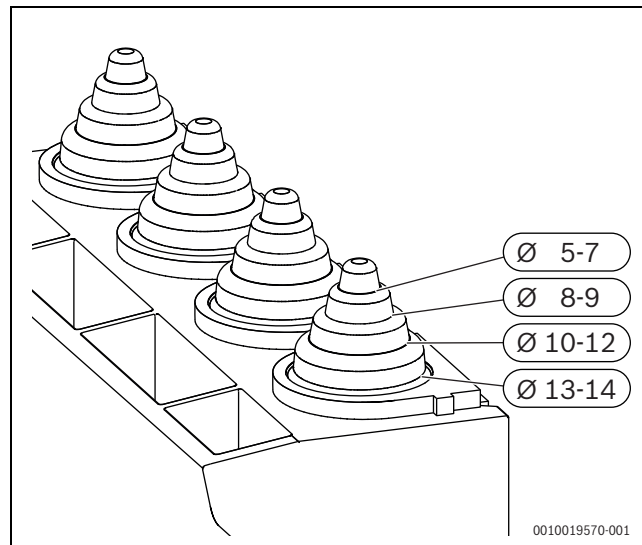
Fig. 30 Adaptar o dispositivo de redução de tração ao diâmetro do cabo
