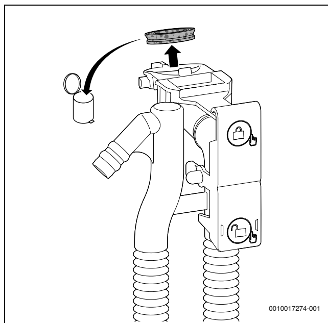
Fig. 57 Retirar a vedação no cimo do sifão de condensados
