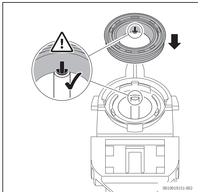
Fig. 58 Alinhar corretamente a nova vedação na recolha de condensados
