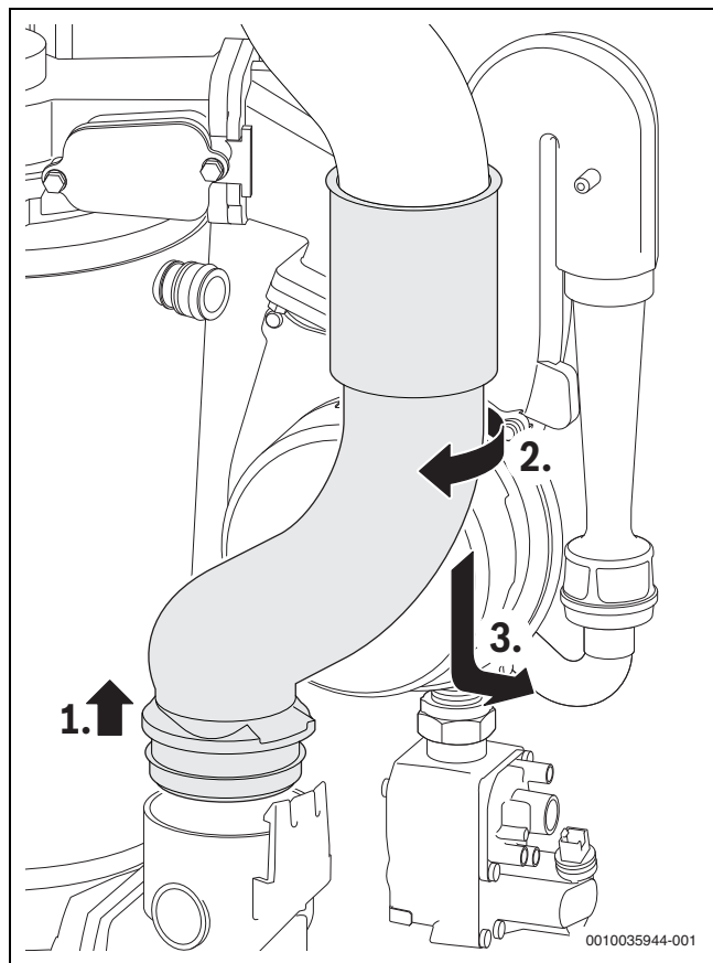
Fig. 43 Desmontar conduta dos gases queimados
