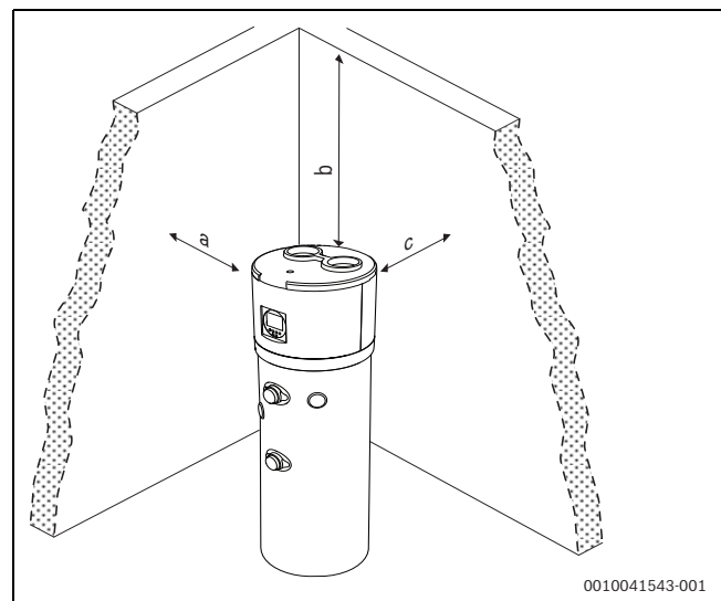
Fig. 9 Distâncias mínimas recomendadas (mm)
