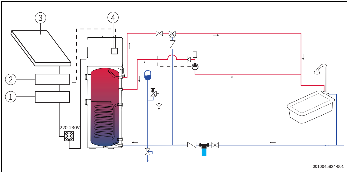
Fig. 37 Recirculação
