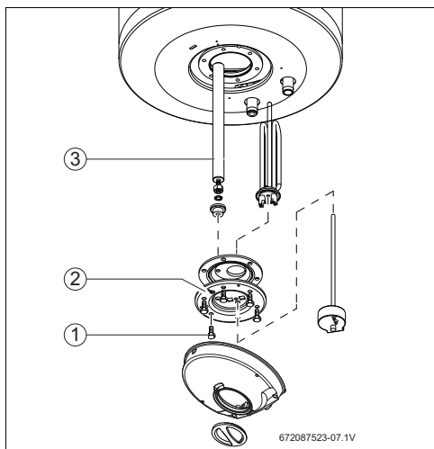
Fig. 15 Acceso a la zona interior e identificación de las partes
