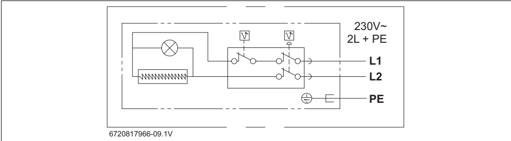
Fig. 17 Esquema de conexiones
