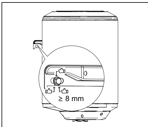
Fig. 11 Instalação vertical (montagem mural)
