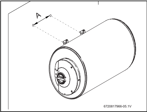
Fig. 12 Instalação horizontal
