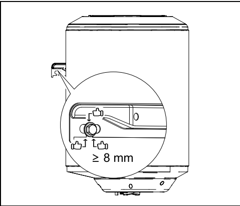
Fig. 11 Instalación en posición vertical
