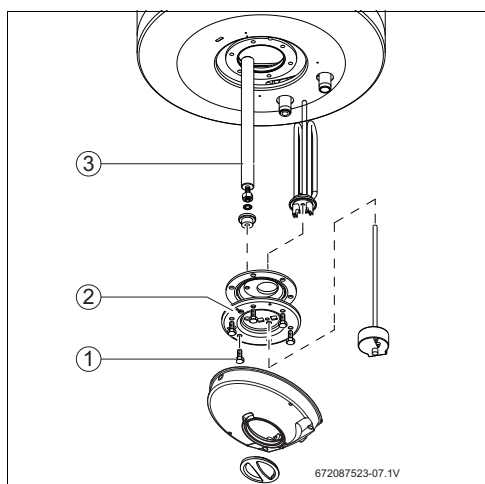
Fig. 15 Accesso a la zona interior e identificación de las par-
