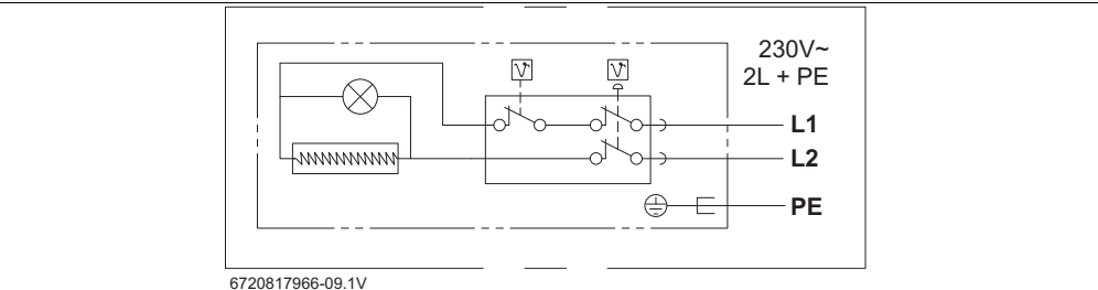
Fig. 17 Schema elettrico di collegamento
