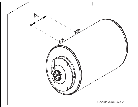
Fig. 12 Instalación en posición horizontal
