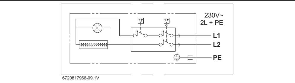
Fig. 17 Esquema de ligação
