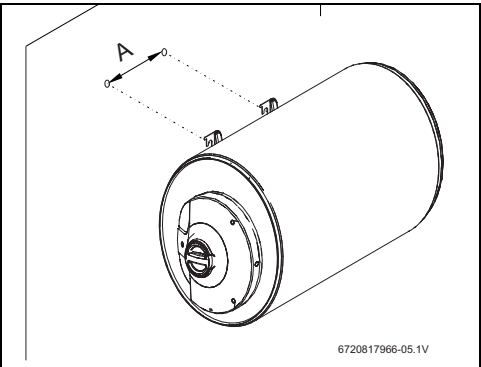
Fig. 12 Instalación en posición horizontal
