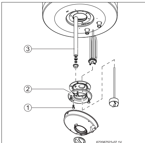
Fig. 15 Acesso e identificação dos componentes internos
