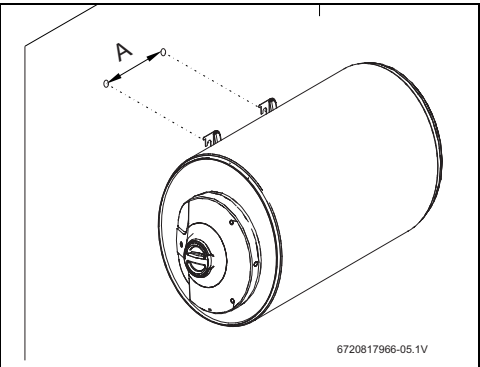
Fig. 12 Installazione orizzontale
