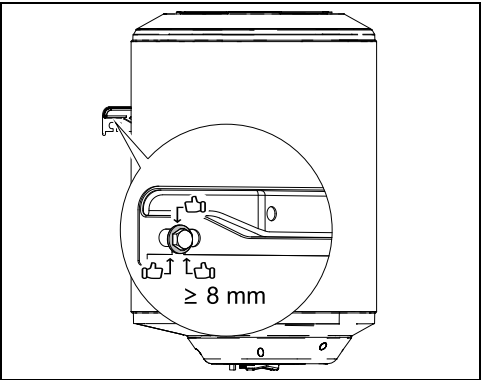
Fig. 11 Instalación en posición vertical
