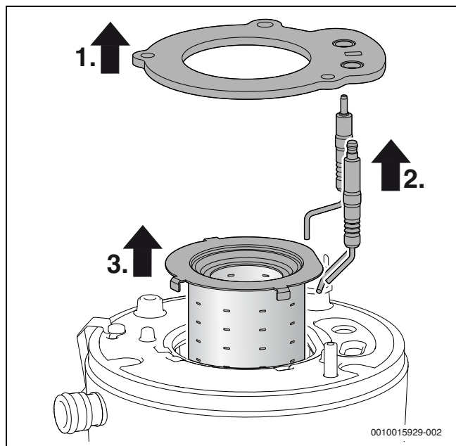
Fig. 43 Retirar o queimador
