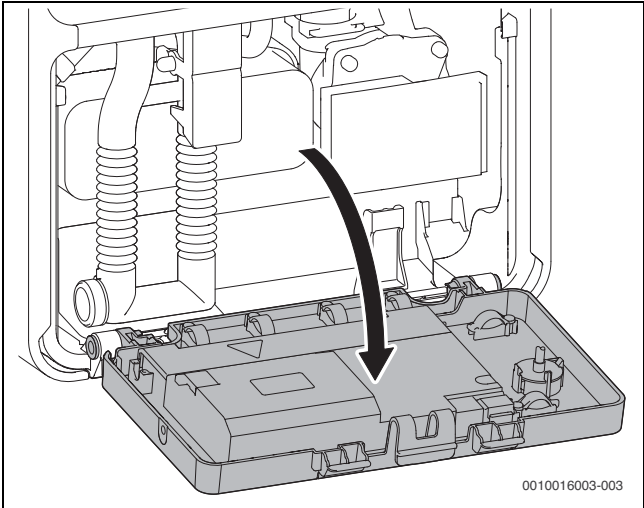
Fig. 25 Inclinar o sistema eletrónico para baixo
