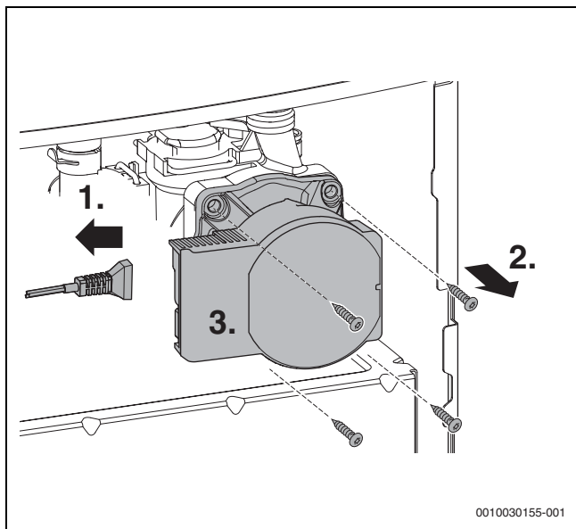
Fig. 60 Desmontar a bomba circuladora
