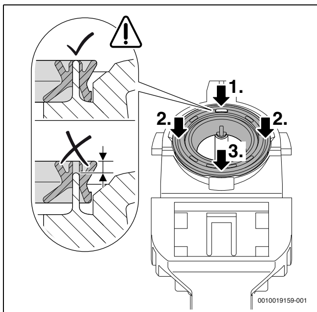
Fig. 53 Pressionar a vedação
