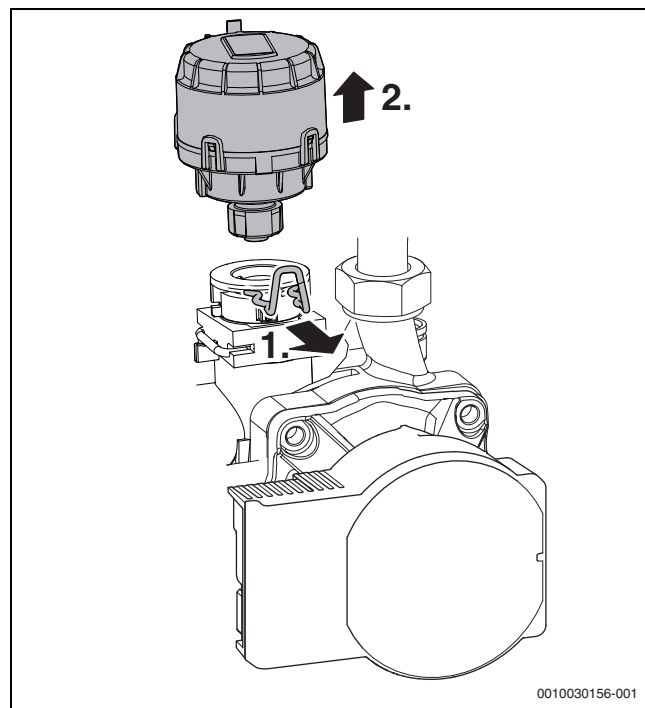
Fig. 62 Desmontar o motor da válvula de 3 vias
