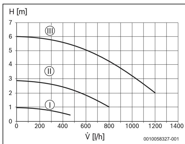
Fig. 32 Curva característica da bomba circuladora (pressão constante)
