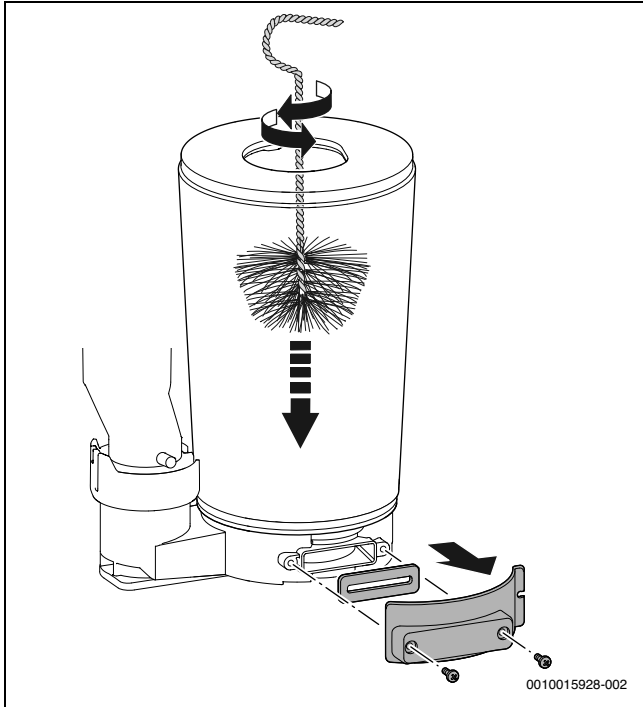
Fig. 46 Limpar o bloco térmico
