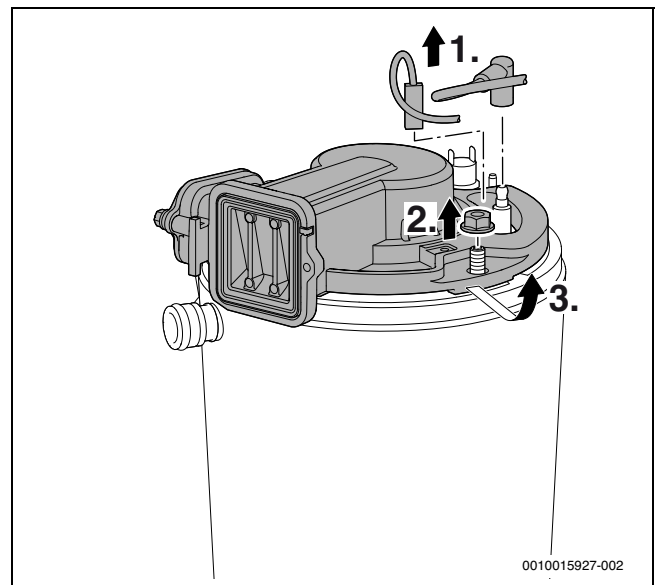
Fig. 41 Soltar a tampa do queimador
