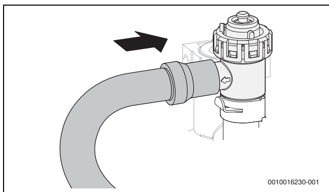
Fig. 22 Instalar a mangueira na válvula de segurança
