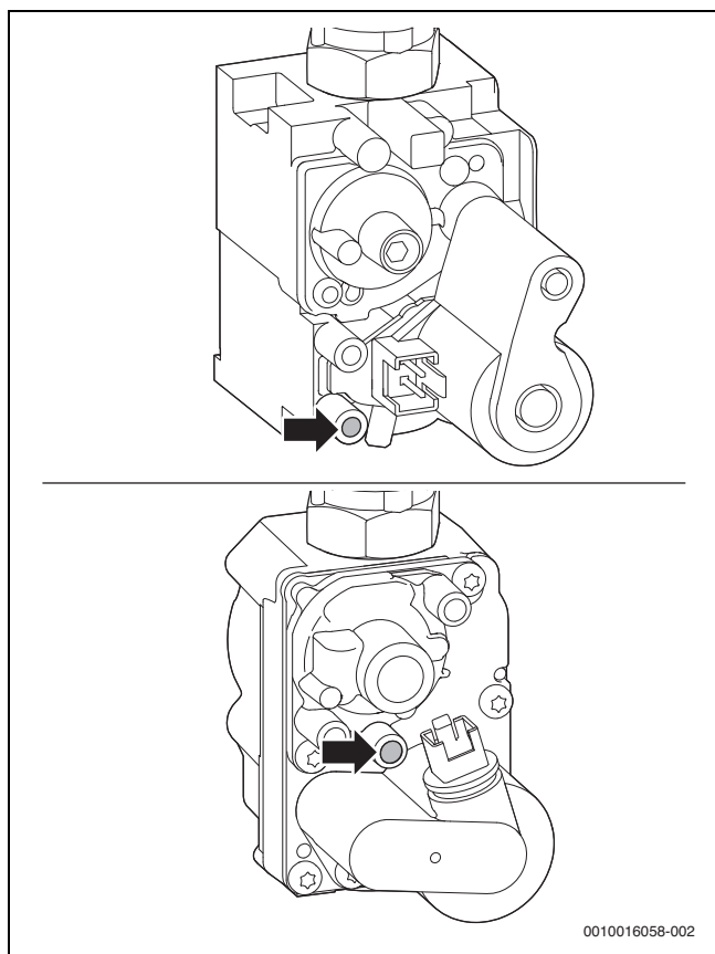
Fig. 37 Ponto de medição para a pressão da ligação de gás
