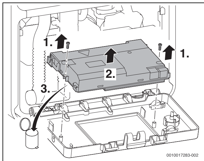
Fig. 65 Substituir o sistema eletrônico do aparelho
