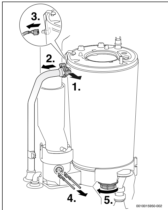
Fig. 63 Soltar o tubo de avanço e retirar o cabo
