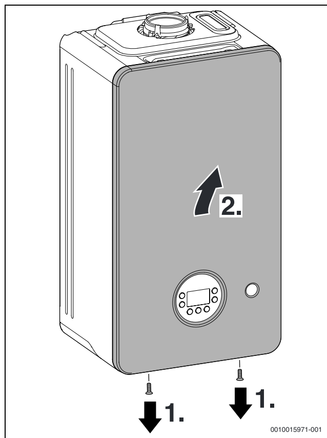
Fig. 21 Retirar o revestimento frontal
