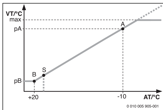
Fig. 71 Curva de aquecimento
