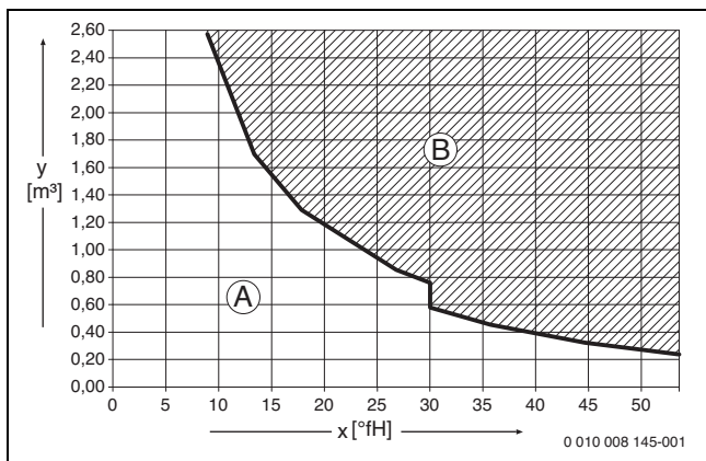
Fig. 19 Requisitos relativos à água de enchimento e à água adicional em °fH para instalações < 50 kW
