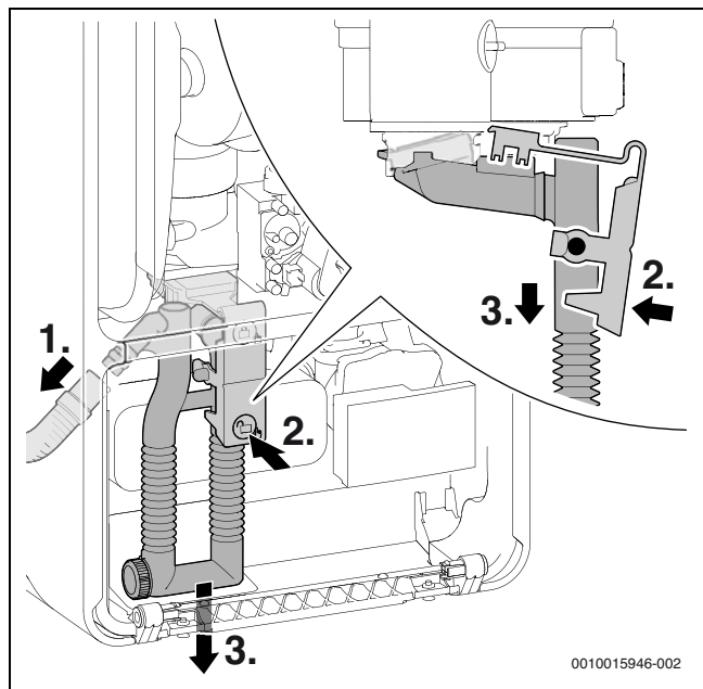
Fig. 49 Desmontar a recolha de condensados
