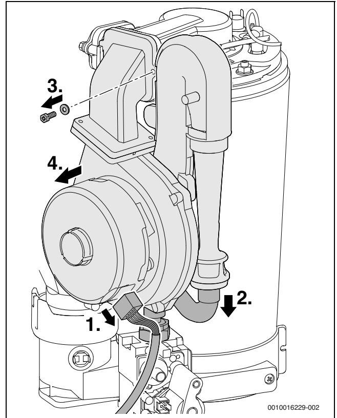
Fig. 40 Desmontar o ventilador com dispositivo de mistura
