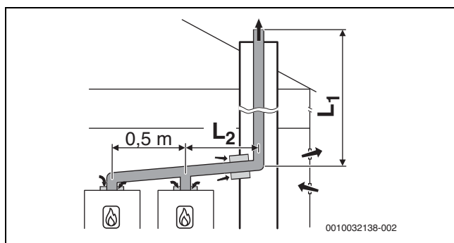
Fig. 17 Cascata com 2 aparelhos: Condução de gases queimados na conduta de acordo com B 23p /B 53p com ar de admissão dependente do ar ambiente no aparelho
