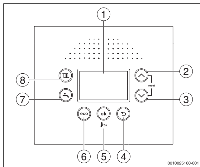
Fig. 28 Vista geral do painel de comando
