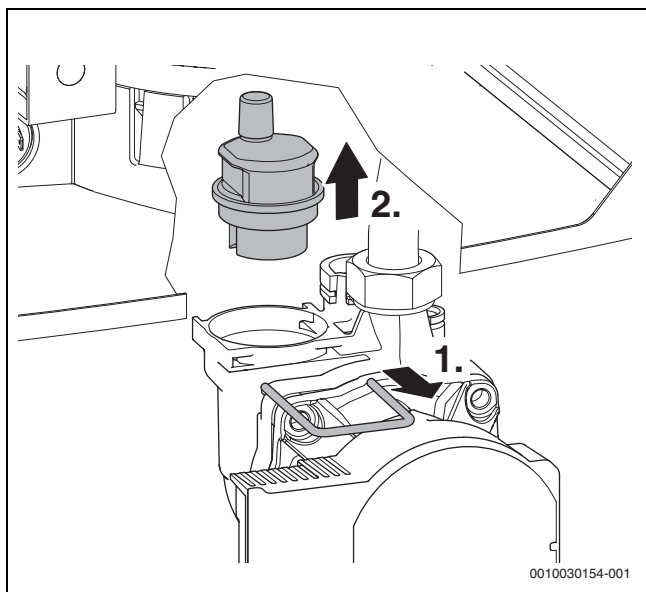
Fig. 61 Desmontar o purgador automático
