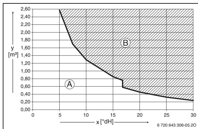
Fig. 18 Requisitos relativos à água de enchimento e à água adicional em °dH para instalações < 50 kW
