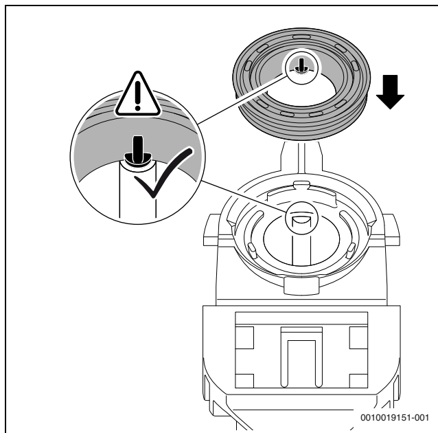
Fig. 52 Alinhar corretamente a nova vedação na recolha de condensados
