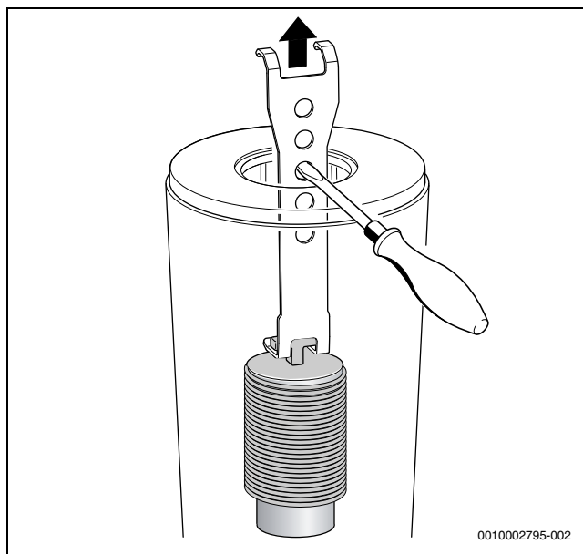
Fig. 45 Retirar o corpo de deslocamento inferior
