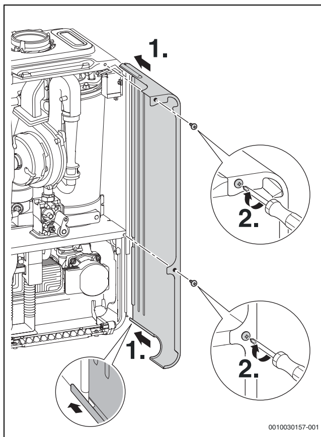
Fig. 67 Montar o revestimento lateral
