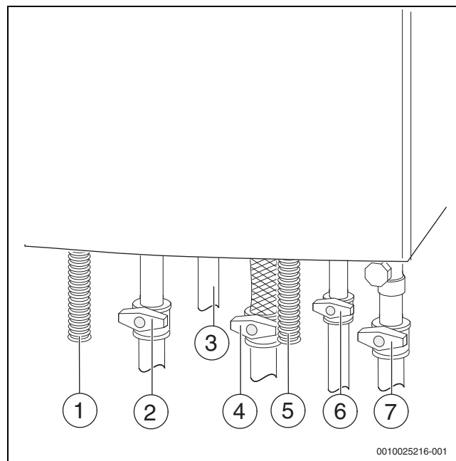
Fig. 24 Ligações do lado do gás e da água (acessórios)
