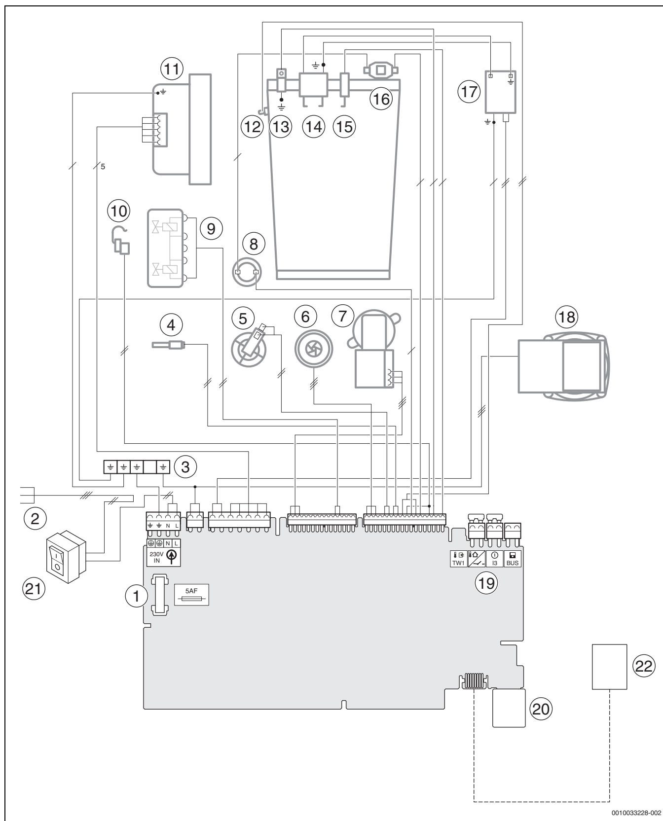
Fig. 70 Cablagem elétrica
