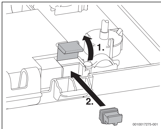
Fig. 66 Inserir a ficha de codificação
