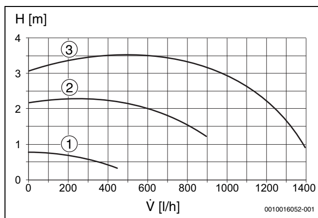
Fig. 33 Curva característica da bomba circuladora (pressão proporcional)
