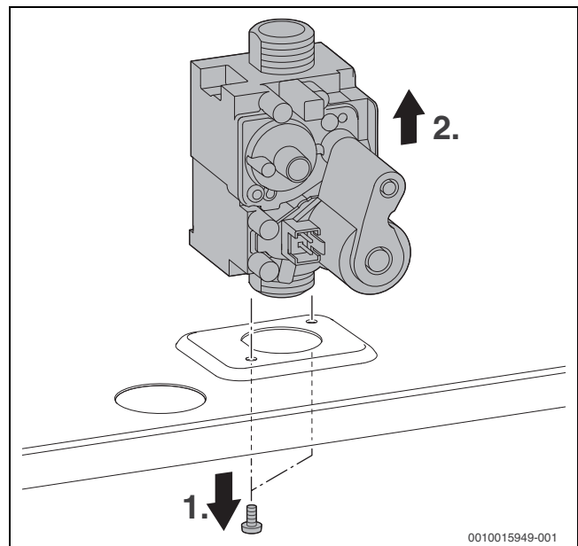
Fig. 59 Desmontar o dispositivo de controlo do gás
