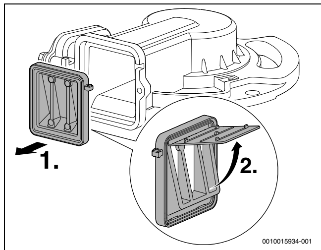
Fig. 42 Válvula antirretorno no dispositivo de mistura
