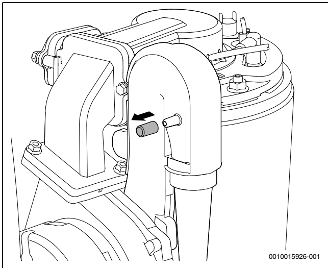
Fig. 39 Ponto de medição no dispositivo de mistura
