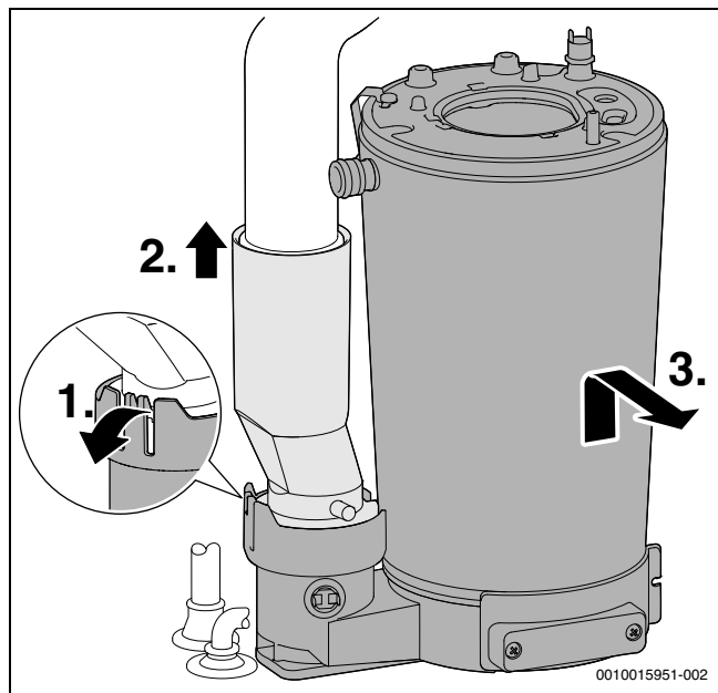
Fig. 64 Desmontar o bloco térmico
