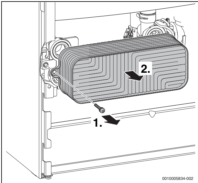
Fig. 57 Desmontar o permutador de calor de placas
