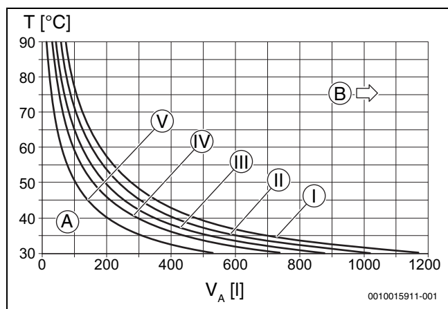
Fig. 20 Curvas características do vaso de expansão
