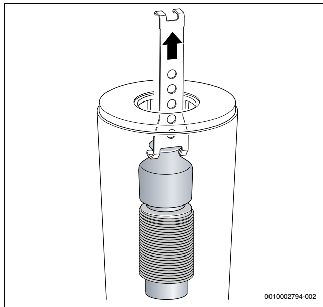
Fig. 44 Retirar o corpo de deslocamento superior
