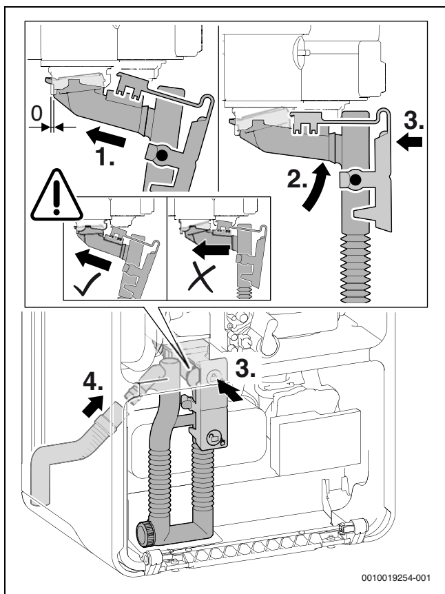
Fig. 54 Instalar a recolha de condensados
