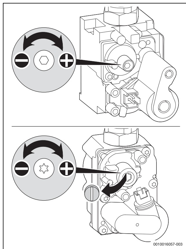
Fig. 35 Retirar o selo de chumbo do parafuso de ajuste
