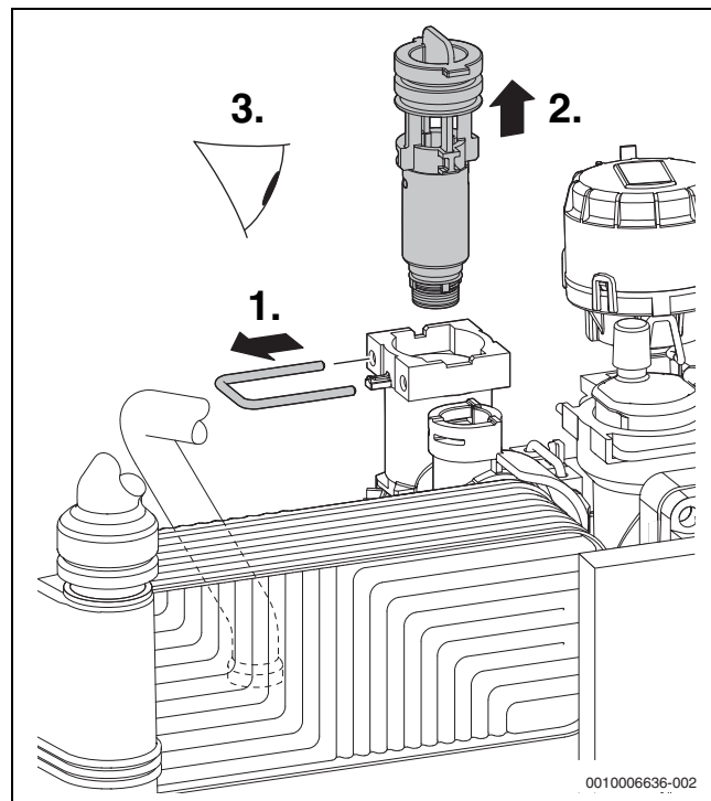
Fig. 56 Verificar o filtro no tubo de água fria
