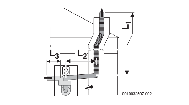
Fig. 12 Encaminhamento de gases queimados de conduta flexível de acordo com C 53 e o sistema de gases queimados com tubos
