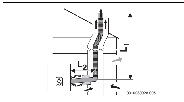
Fig. 16 Tubagem flexível de gases queimados no compartimento de acordo com B 53p com ar de admissão dependente do ar ambiente no aparelho e tubo de gases queimados simples no local de instalação; abertura de ventilação traseira no compartimento
