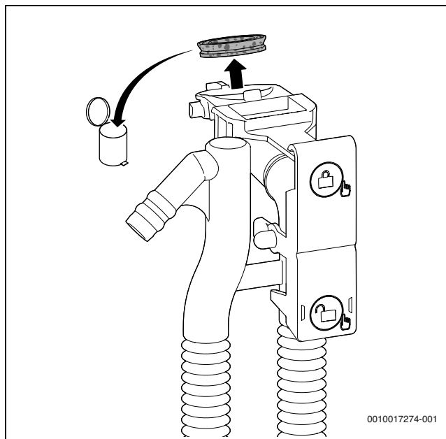
Fig. 51 Retirar a vedação no cimo do sifão de condensados
