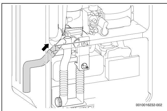
Fig. 23 Montar a mangueira na recolha de condensados
