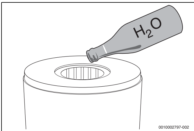
Fig. 48 Lavar o bloco térmico com água
