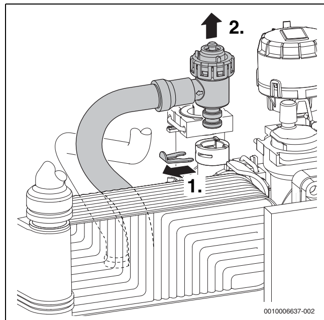
Fig. 55 Retirar a válvula de segurança (circuito de aquecimento)
