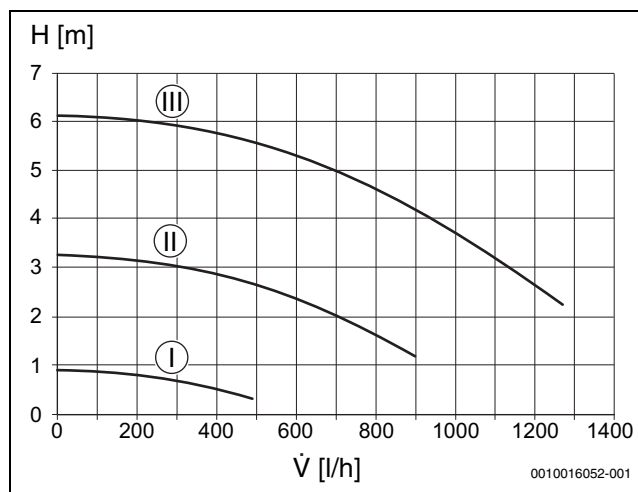
Fig. 31 Curva característica da bomba circuladora (rotações constantes)
