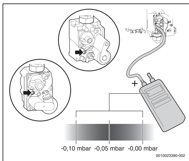
Fig. 34 Inspeção da pressão diferencial
