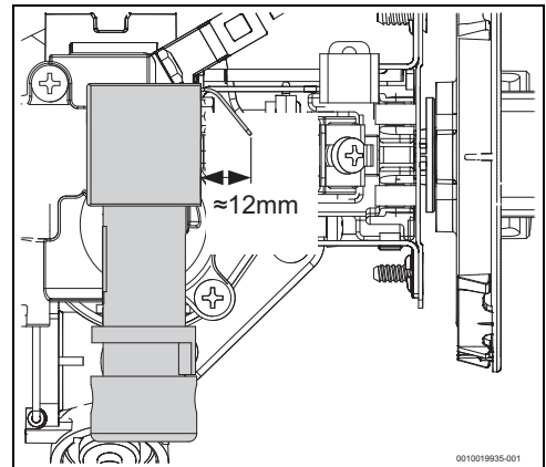
Fig. 24 Posição do arame de contacto
