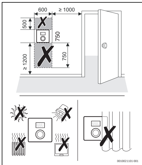
Fig. 5 Loca de instalação Unidade de comando
