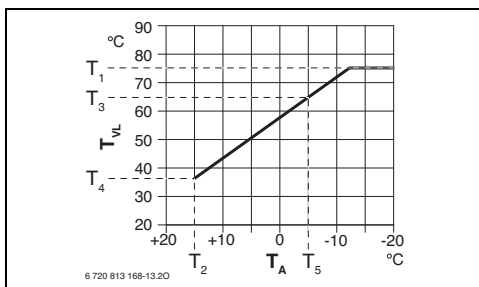
Fig. 14 Esquema de aquecimento para um sistema de aquecimento com radiadores convencionais
