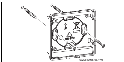
Fig. 8 Instalar o caixilho da parede da unidade de comando
