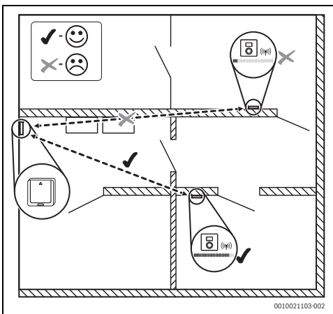
Fig. 6 Ligações via rádio
