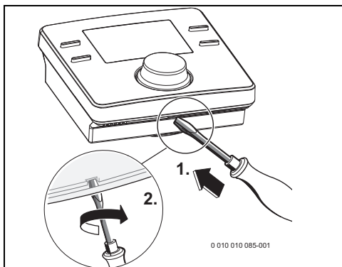
Fig. 7 Retirar a unidade de comando do caixilho da parede
