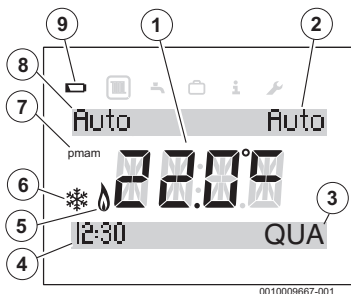
Fig. 9 Vista padrão do visor
