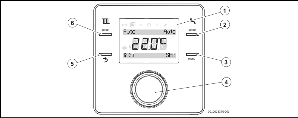
Fig. 1 Unidade de comando
