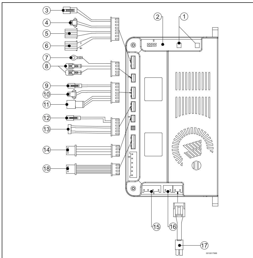
Fig. 29 Esquema elétrico
