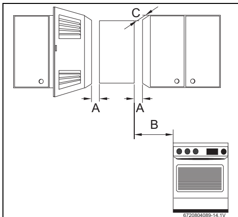
Fig. 20 Distâncias mínimas
