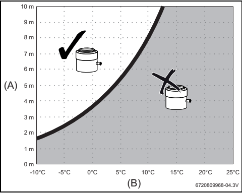
Fig. 17 Condutas concêntricas
