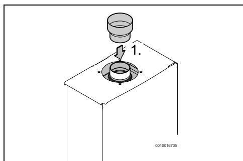
Fig. 23 Montagem do adaptador de exaustão
