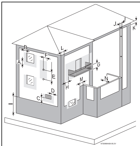
Fig. 21 Distâncias mínimas a pontos de exaustão
