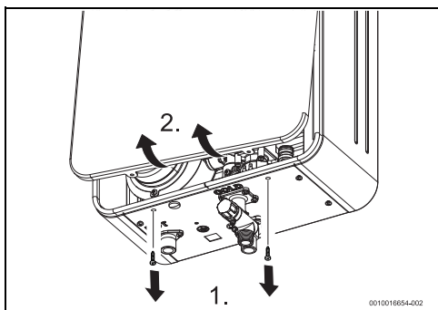
Fig. 27 Retirar a frente
