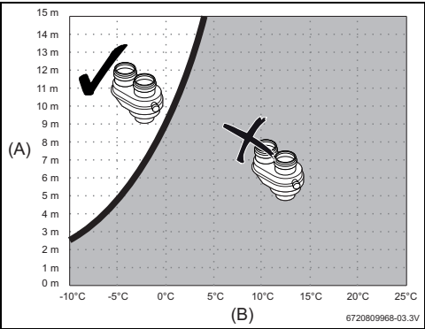
Fig. 18 Condutas separadas
