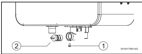
Fig. 16 Purga
