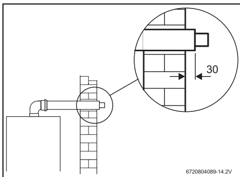
Fig. 25 Dimensões (em mm)
