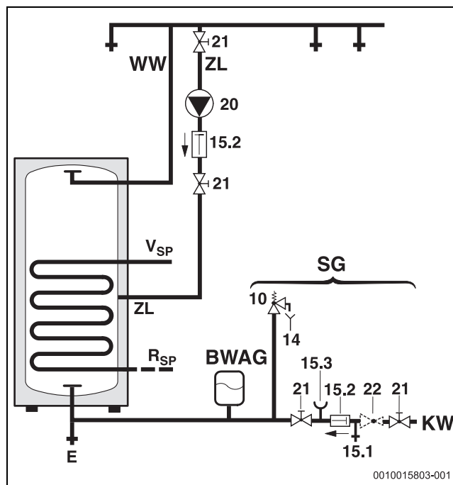
Fig. 2 Schema de racordare la nivelul apei potabile
