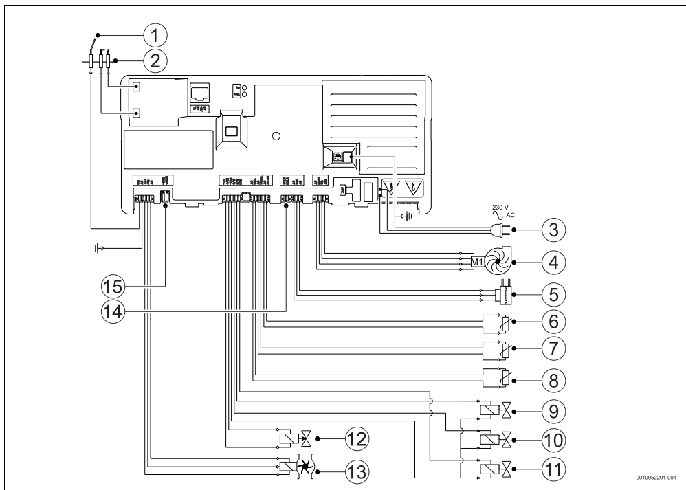
Fig. 32 Esquema elétrico
