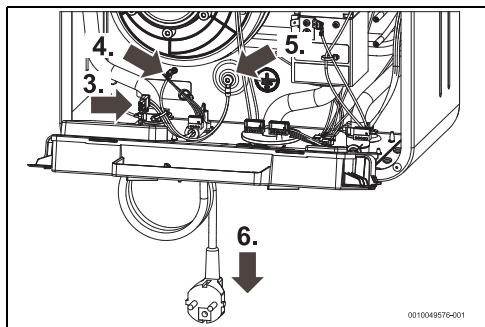
Fig. 28 Ligação do cabo de alimentação
