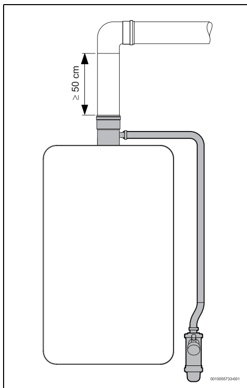
Fig. 17 Recolha de condensados (conduta horizontal)
