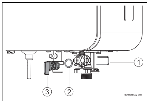
Fig. 15 Purga
