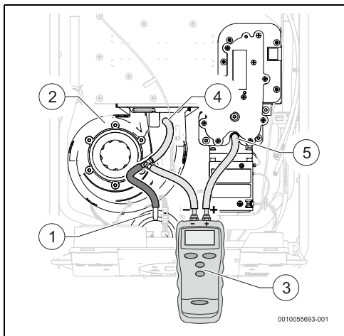
Fig. 29 Ligação ao ventilador, sensor de pressão e tomada de pressão de gás
