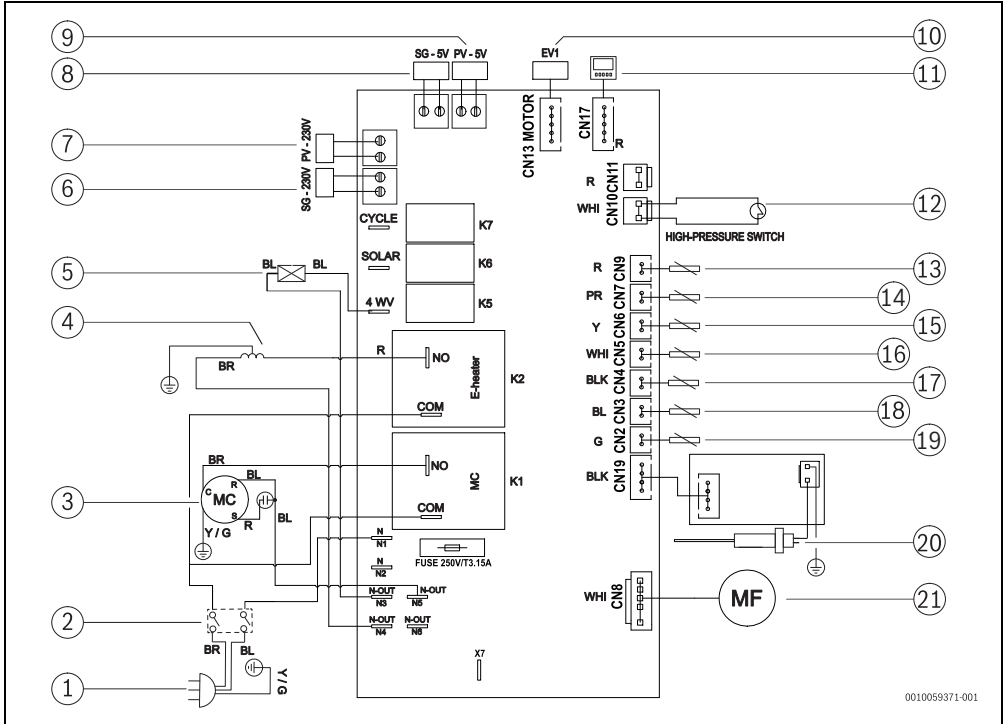
Fig. 27 Esquema eléctrico
