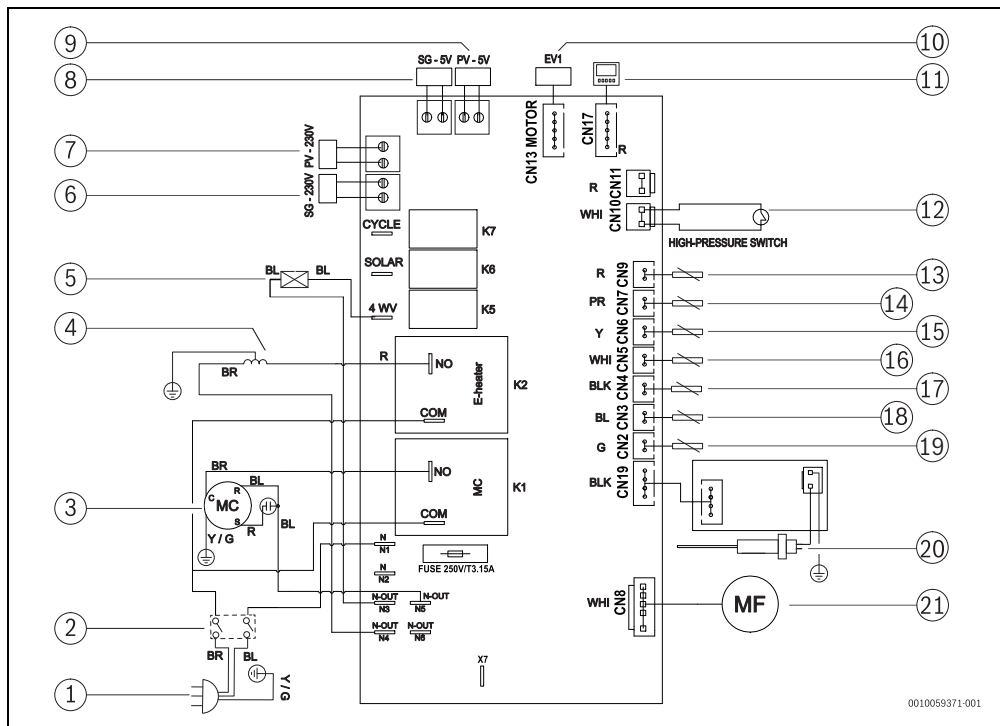
Fig. 27 Schema elettrico
