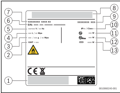
Fig. 2 Descripción de la placa de características
