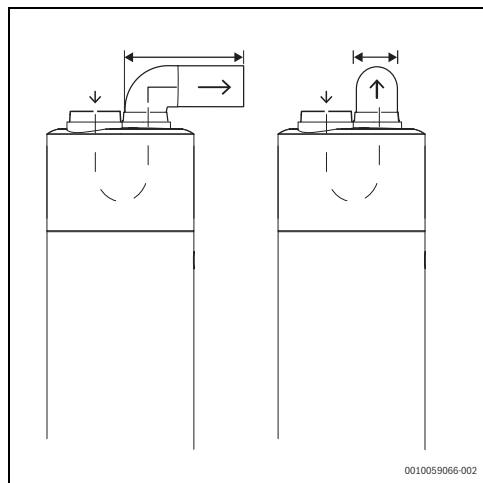
Fig. 10 Conducto de aire específico
