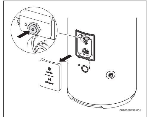
Fig. 26 Resetear el termostato de seguridad
