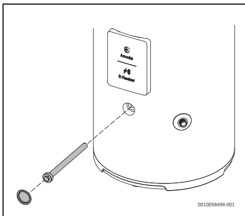
Fig. 25 Desmontaje del ánodo de magnesio
