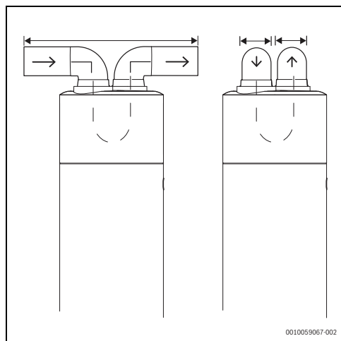
Fig. 11 Segundo canal de ventilación específico
