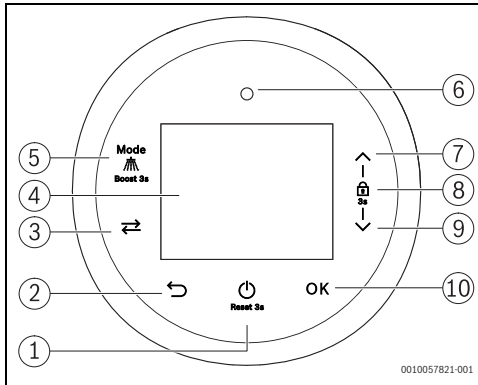
Fig. 18 Panel de mando
