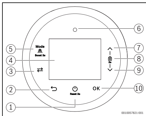
Fig. 24 Panel de mando
