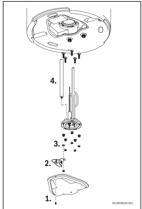
Fig. 31 Remoção do ânodo de magnésio
