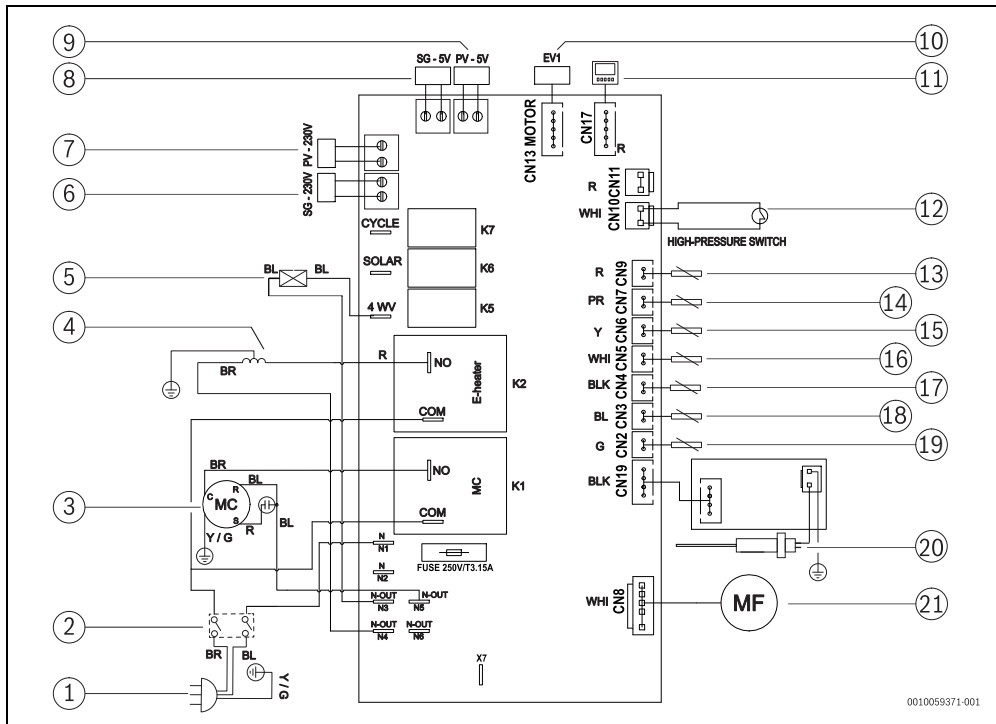
Fig. 33 Esquema eléctrico
