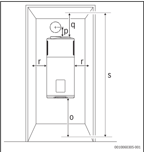
Fig. 9 Distancias mínimas sin estructura de apoyo
