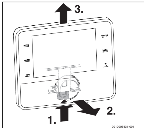
Fig. 5 Retirar a unidade de comando
