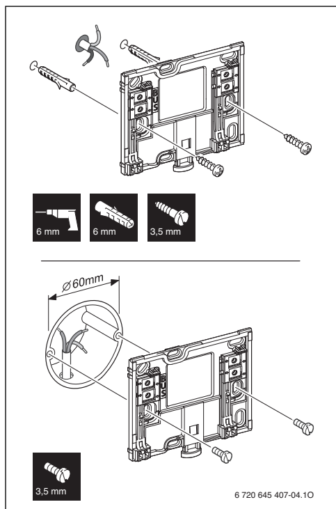
Fig. 3 Instalação da base
