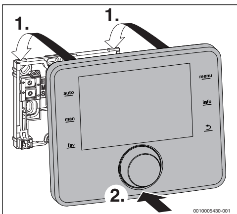
Fig. 4 Encaixar a unidade de comando
