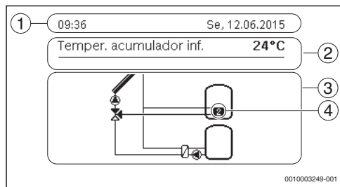
Fig. 2 Exemplo dos símbolos na indicação padrão
