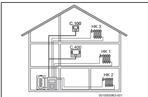
Fig. 2 Exemplo de instalação de aquecimento com três circuitos de aquecimento e CR 100 como comando à distância (habitação unifamiliar com pequeno apartamento para arrendamento ou oficina)
