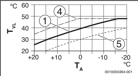
Fig. 13 Ajuste da curva de aquecimento para aquecimento do piso Deslocação paralela acima da temperatura ambiente pretendida
