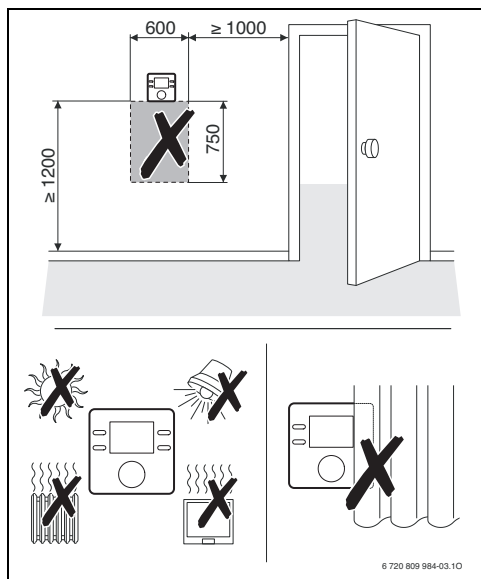
Fig. 6 Local de instalação na zona de referência
