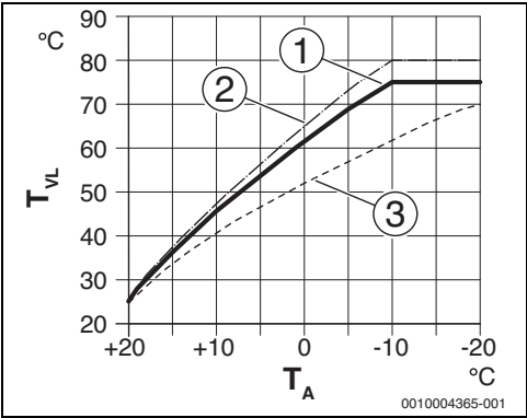
Fig. 14 Ajuste da curva de aquecimento para radiadores Aumento acima da temperatura de projeto T_P e da temperatura exterior mínima T_{E,min}
