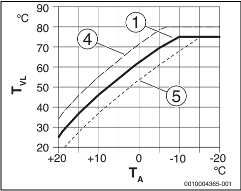
Fig. 15 Ajuste da curva de aquecimento para radiadores Deslocação paralela acima da temperatura ambiente pretendida
