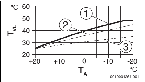
Fig. 11 Ajuste da curva de aquecimento para aquecimento do piso Aumento acima da temperatura de projeto T_P e da temperatura exterior mínima T_{E,min}
