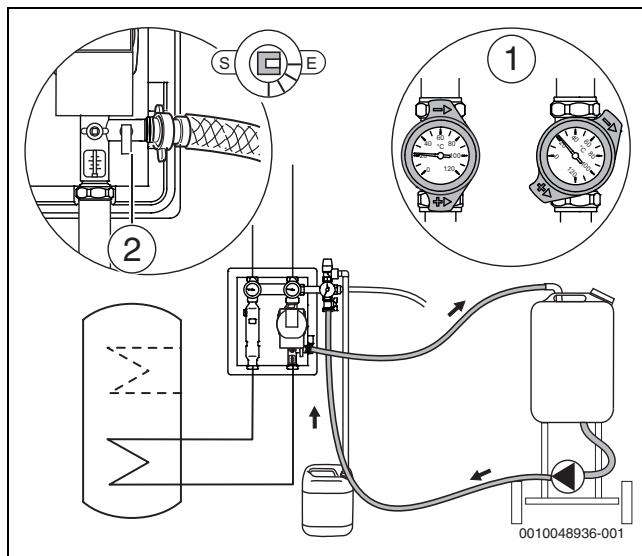
Fig. 36 Purga do sistema padrão
