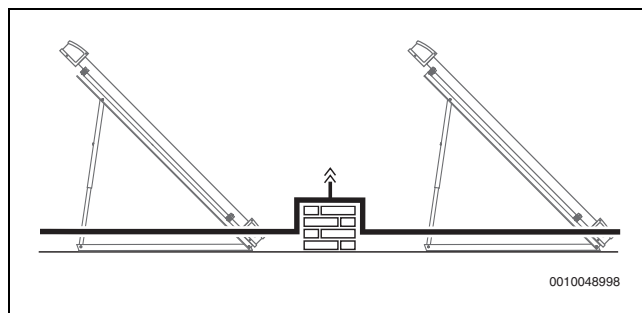
Fig. 11 Várias baterias de coletores ligadas paralelamente com purgador adicional (tubagem de avanço)
