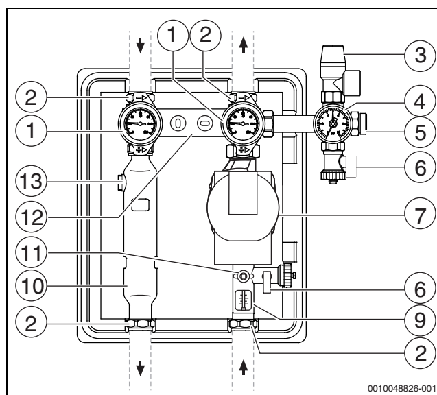
Fig. 3 Grupo de circulação solar de 2 condutas sem peça de isolamento frontal e sem controlador integrado e módulos
