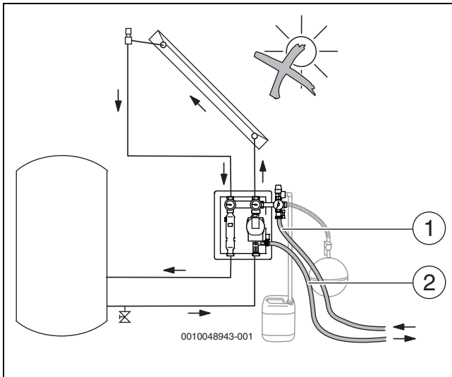
Fig. 39 Grupo de circulação solar com válvulas de esfera e válvula de retenção nos termômetros
