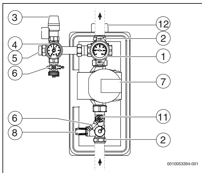
Fig. 2 Grupo de circulação solar de 1 conduta sem isolamento frontal
