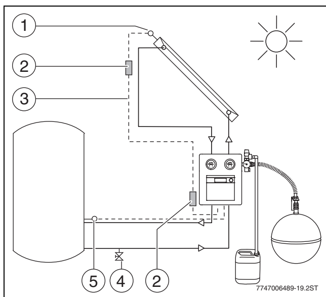
Fig. 25 Sensor de temperatura no grupo de circulação solar com controlador integrado
