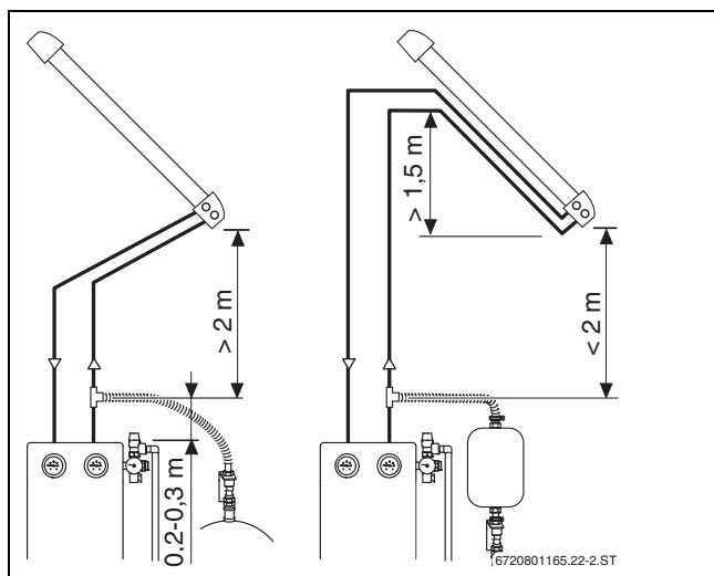
Fig. 15 Distância ao campo de coletores (coletores de tubos de vácuo)
