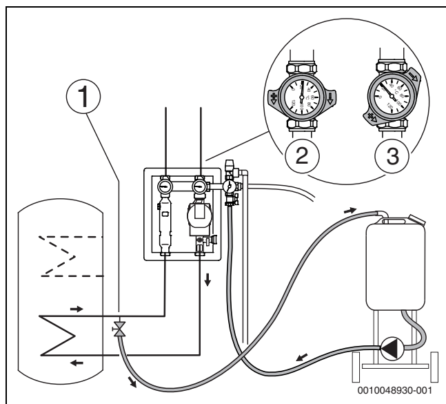
Fig. 27 Purga abaixo do grupo de circulação solar
