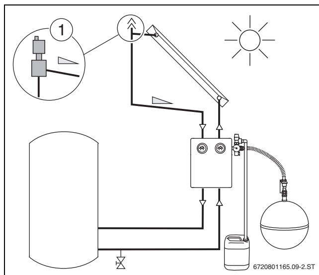
Fig. 12 Posição do purgador automático
