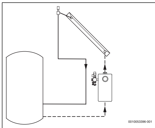
Fig. 7 Sistema padrão com grupo de circulação solar de 1 conduta e purgador no topo do telhado
