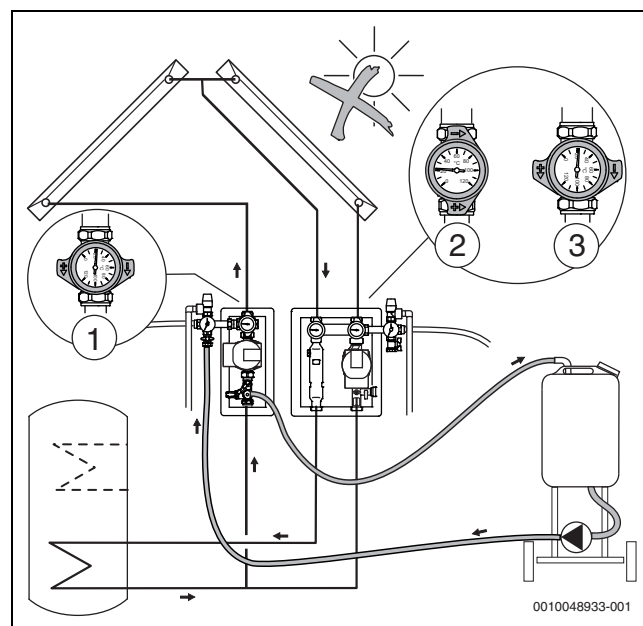
Fig. 33 Purga do campo de coletores esquerdo
