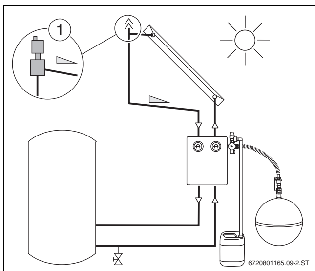
Fig. 16 Posição do purgador automático
