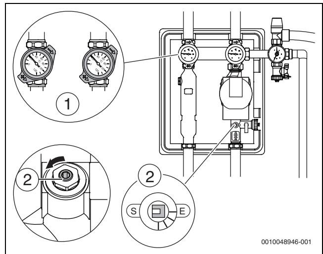
Fig. 42 Válvulas de fecho abertas
