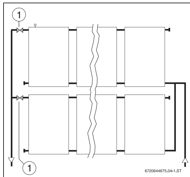
Fig. 32 Purga de campo de coletores ligados em paralelo
