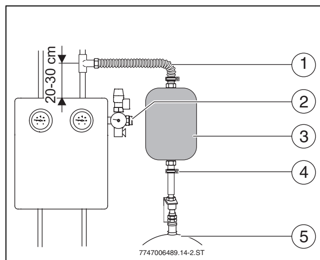
Fig. 22 Montagem do vaso auxiliar
