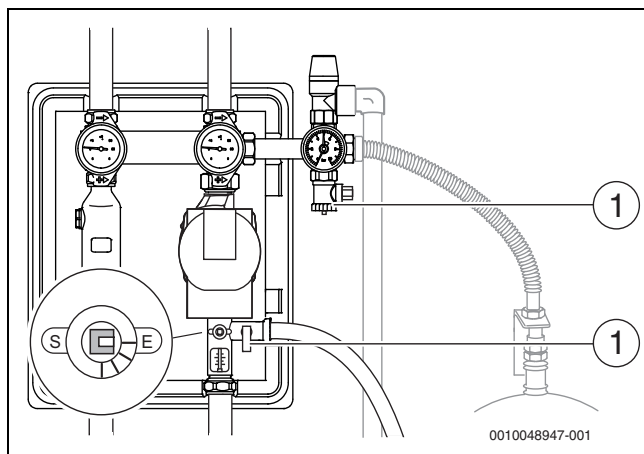
Fig. 43 Enchimento através da válvula da torneira de enchimento e drenagem
