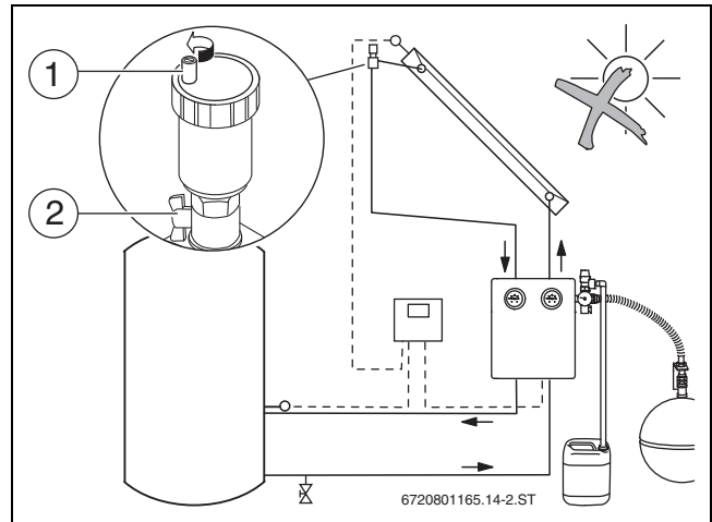
Fig. 41 Abrir o purgador
