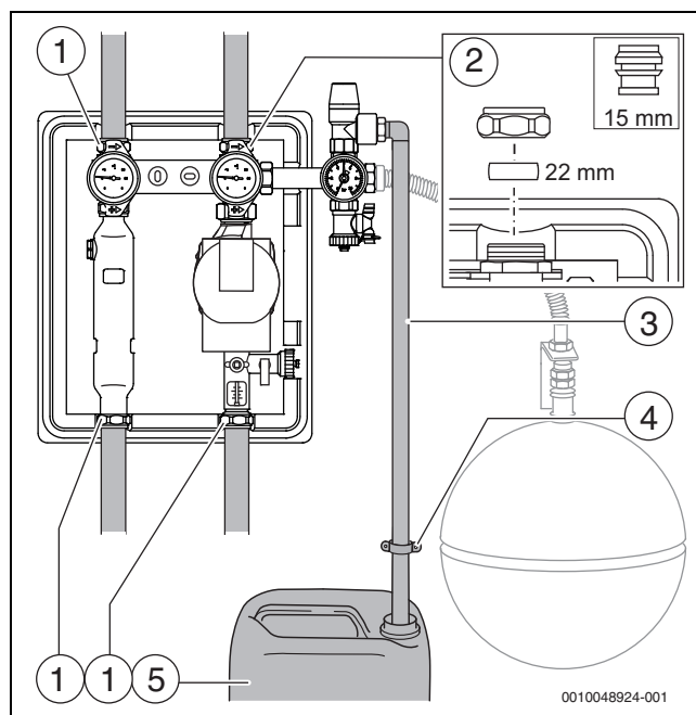
Fig. 24 Ligação ao grupo de circulação solar
