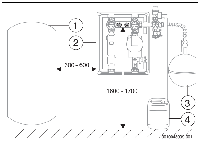
Fig. 19 Colocação recomendada (medida em mm)
