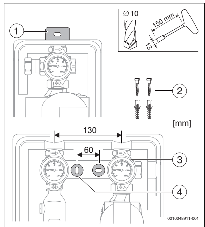
Fig. 20 Montagem do grupo
