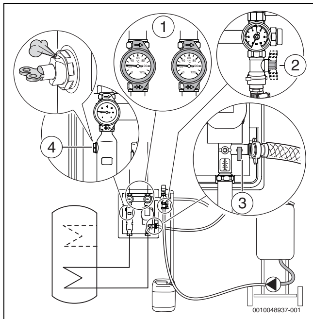
Fig. 37 Fechar e abrir torneiras de enchimento e drenagem
