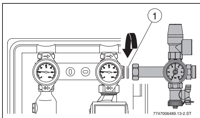
Fig. 21 Montar o grupo de segurança
