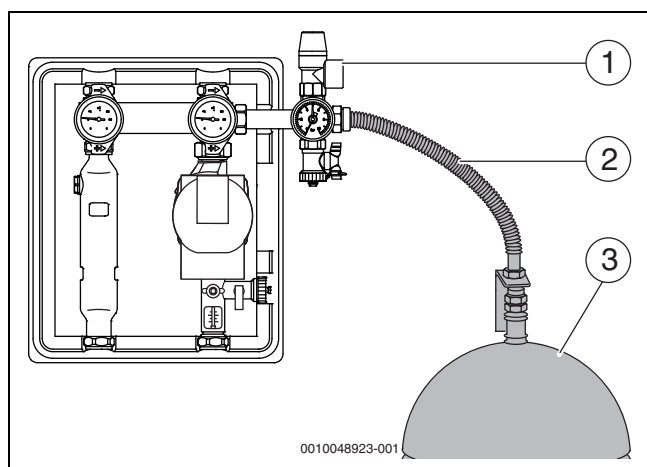
Fig. 23 Montagem dos vasos de expansão
