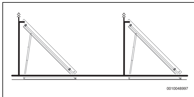
Fig. 13 Várias baterias de coletores ligadas paralelamente com purgadores adicionais (tubagem de avanço)
