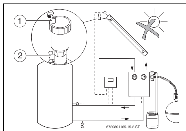
Fig. 45 Fechar o purgador e a válvula de esfera
