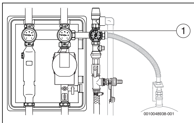
Fig. 44 Verificar o visor do manômetro
