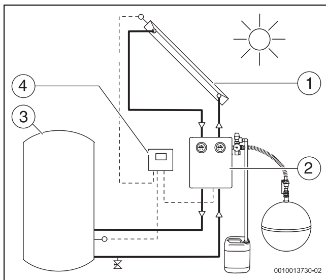
Fig. 8 Representação de exemplo de uma instalação de energia solar
