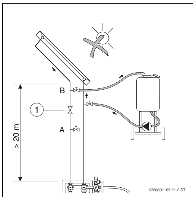
Fig. 29 Purgar a parte superior do sistema
