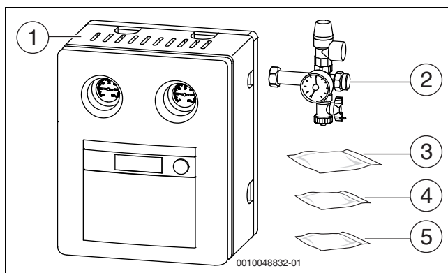
Fig. 9 Grupo de circulação solar, aqui: com controlador integrado
