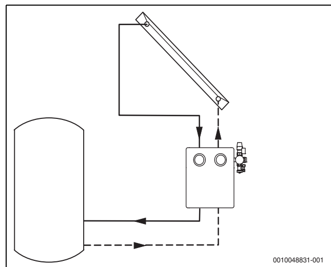
Fig. 4 Sistema padrão com grupo de circulação solar de 2 condutas
