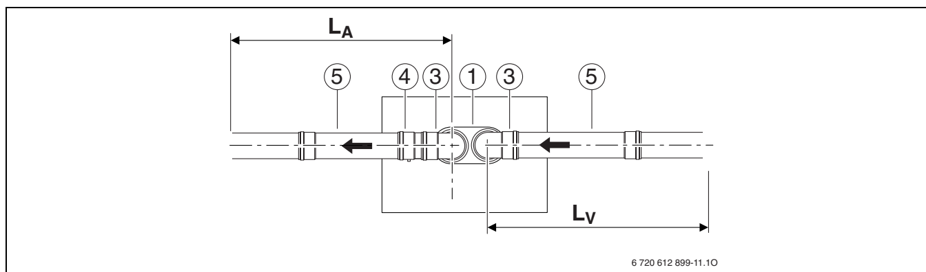
Fig. 13 Conduta de gases de combustão conforme C 42 , C 52 e C 82
