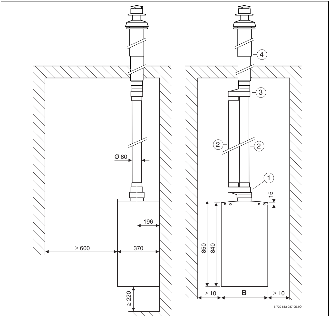
Fig. 10 Conduto de exaustão-admissão conforme C 32
