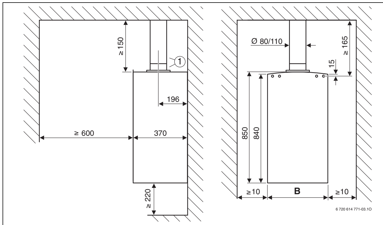
Fig. 4 Tecto plano
