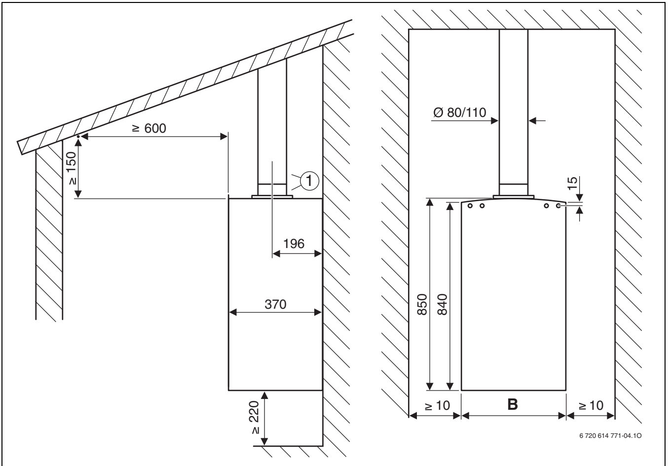
Fig. 5 Tecto inclinado
