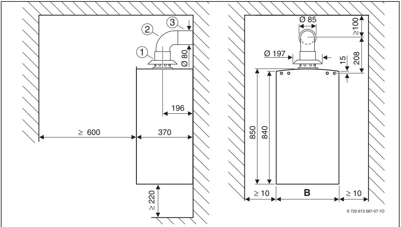
Fig. 2 Sistema de exaustão de gases queimados conforme B 22
